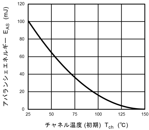
アバランシェエネルギー E_{AS} (mJ) チャンネル温度 (初期) T_{ch} (°C) 図 8.14 E_{AS} - T_{ch} (最大値 (保証値))
