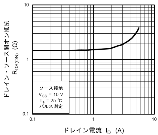
図 8.6 R_{DS(\text{ON})} - I_D
