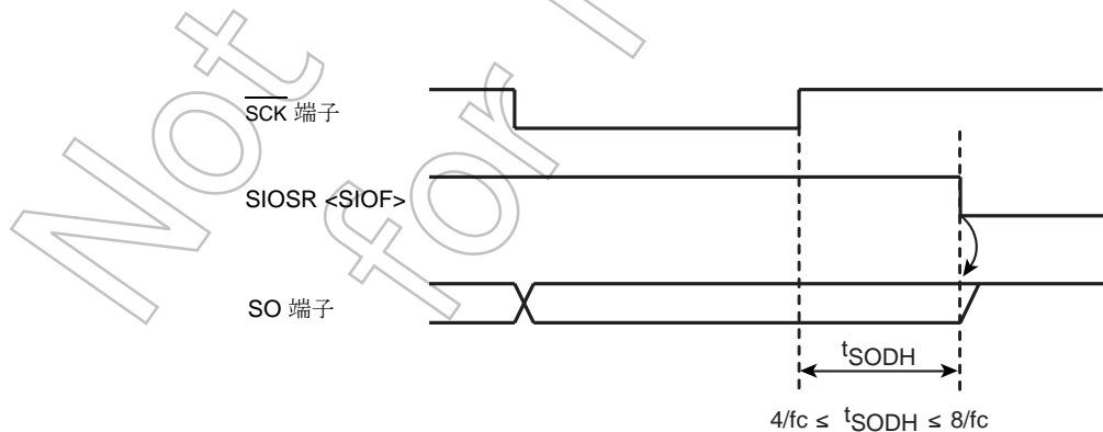
図 10-17 送受信終了時のデータ保持時間
