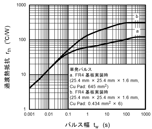
図 7.10 r_{th} - t_w
