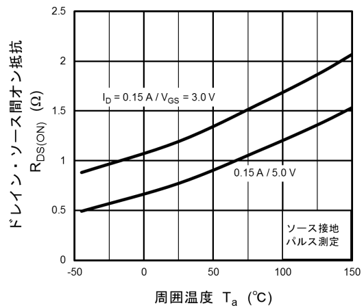
図 7.6 R_{DS(ON)} - T_a
