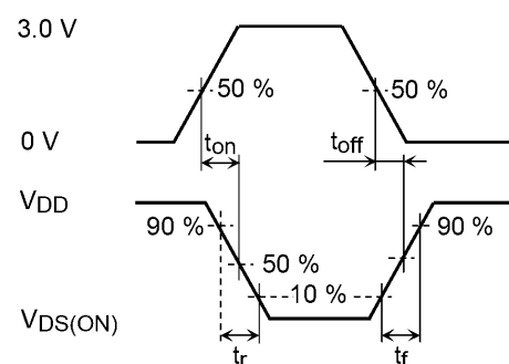
図 5.3.2 入力波形/出力波形
