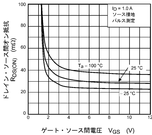
図 8.3 R_{DS(ON)} - V_{GS}
