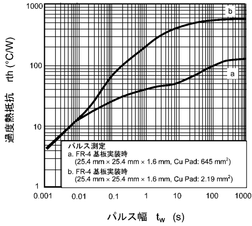
図 9.13 r_{th} - t_w
