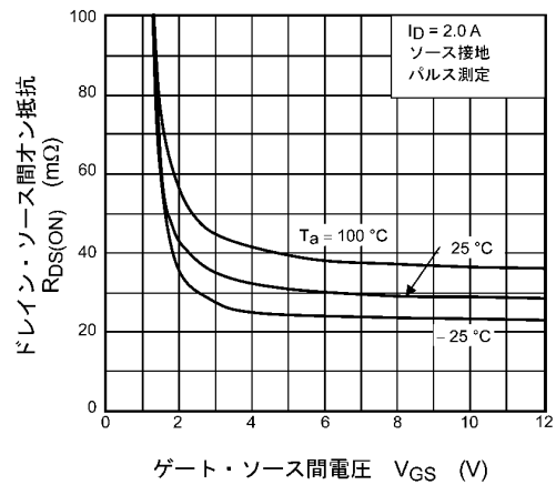
図 8.4 R_{DS(ON)} - V_{GS}
