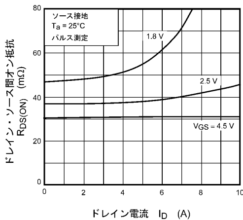
図 8.5 R_{DS(ON)} - I_D
