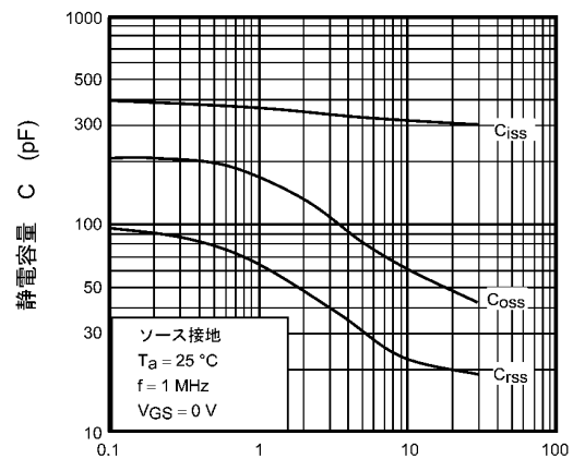
図 9.10 C - V_{DS}
