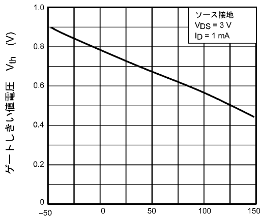
図 9.7 V_{th} - T_a
