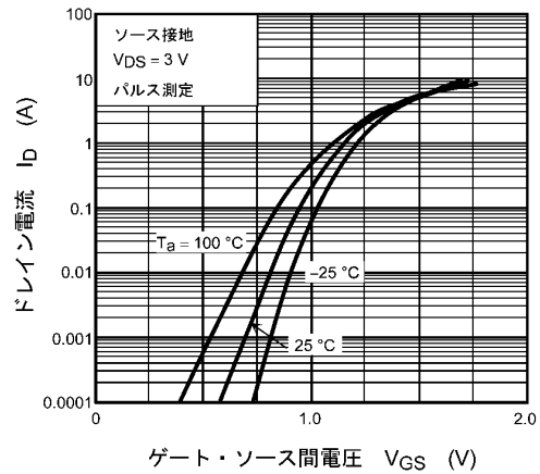
図 8.2 I_D - V_{GS}
