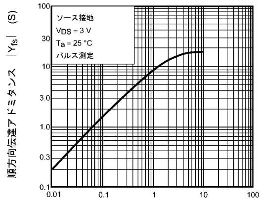
図 9.8 |Y_{fs}| - I_D
