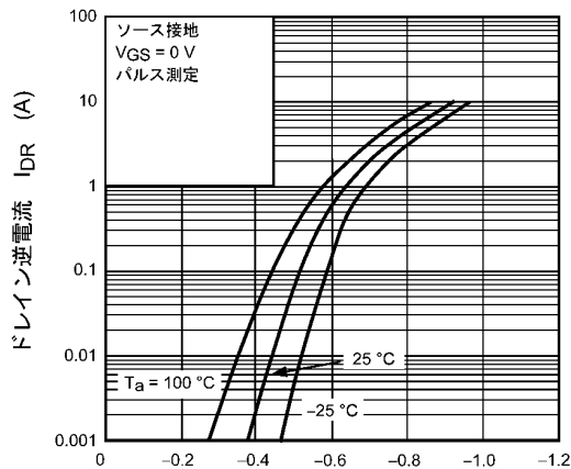
図 9.9 I_{DR} - V_{DS}
