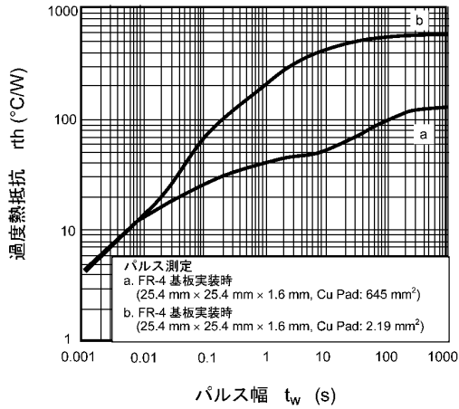
図 8.13 r_{th} - t_w
