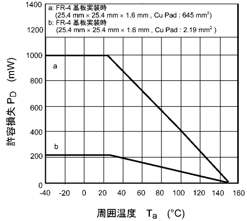
図 8.14 P_D - T_a
