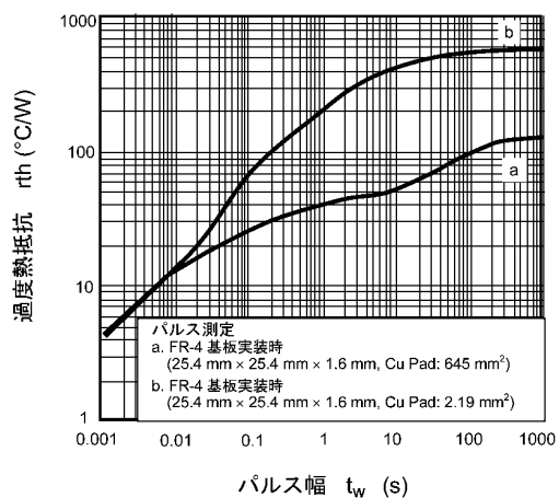
図 8.13 r_{th} - t_w
