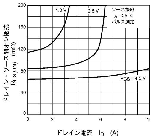
図 8.5 R_{DS(ON)} - I_D
