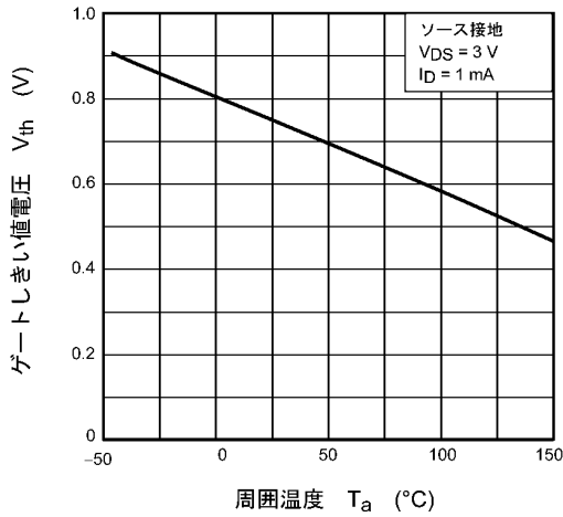
図 8.7 V_{th} - T_a
