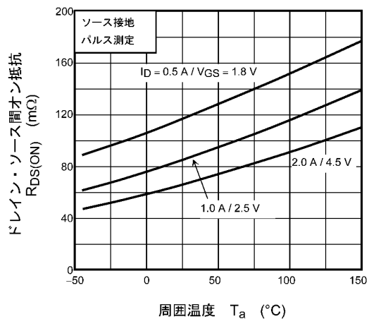
図 8.6 R_{DS(ON)} - T_a
