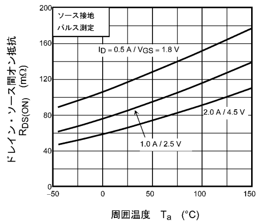
図 8.6 R_{DS(ON)} - T_a
