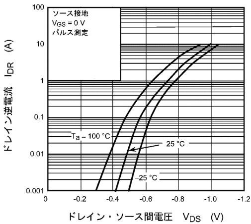
図 9.9 I_{DR} - V_{DS}
