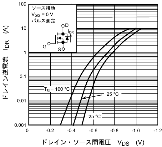
図 8.9 I_{DR} - V_{DS}
