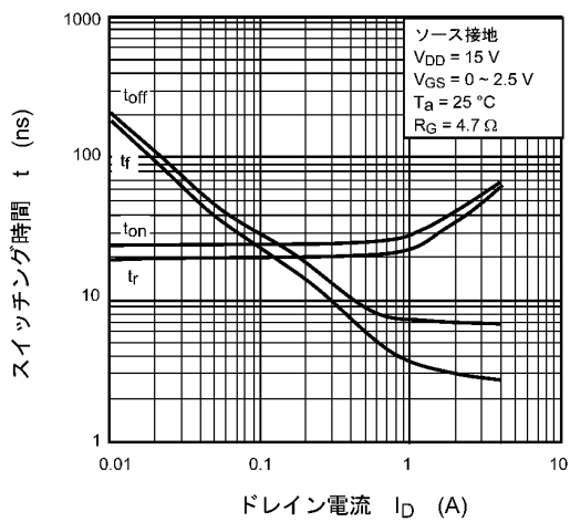
図 8.11 t - I_D
