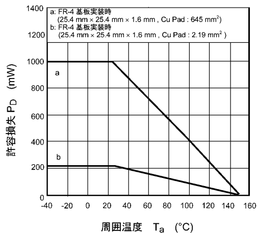
図 8.14 P_D - T_a
