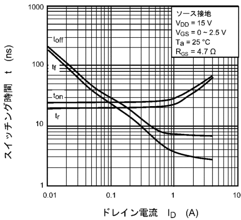
図 9.11 t - I_D
