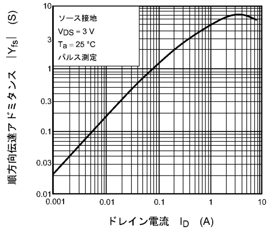
図 9.8 |Y_{fs}| - I_D
