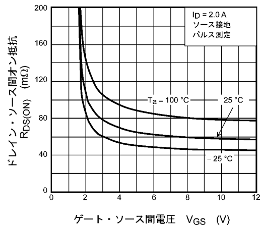
図 8.4 R_{DS(ON)} - V_{GS}
