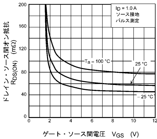
図 9.3 R_{DS(ON)} - V_{GS}
