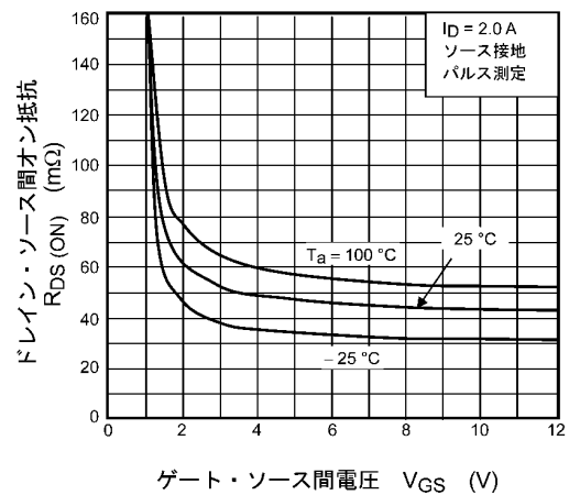
図 7.4 R_{DS(ON)} - V_{GS}
