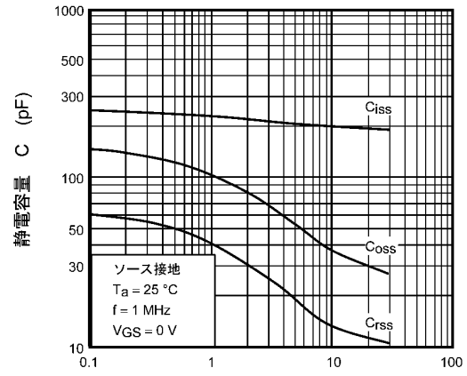
図 7.10 C - V_{DS}
