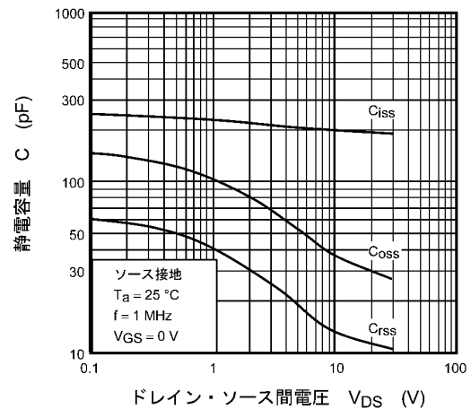
図 9.10 C - V_{DS}
