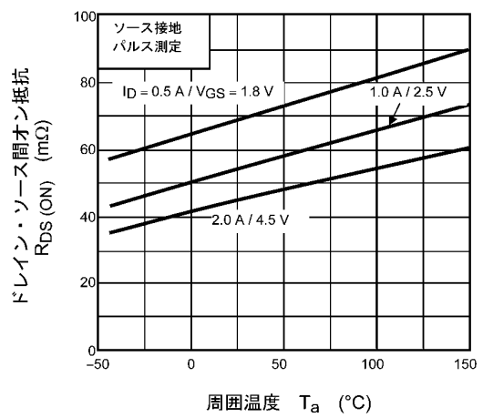
図 7.6 R_{DS(ON)} - T_a
