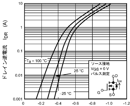
図 7.9 I_{DR} - V_{DS}
