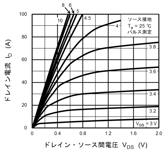
図 8.2 I_D - V_{DS}
