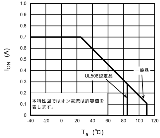
図 14.1.2 I_{ON} - T_a
