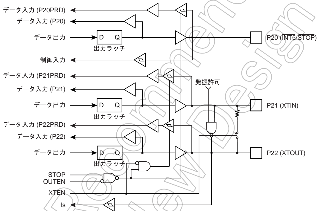
図 5-4 P2 ポート
