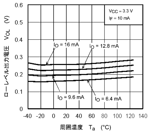
図 12.2.4 V_{OL} - T_a
