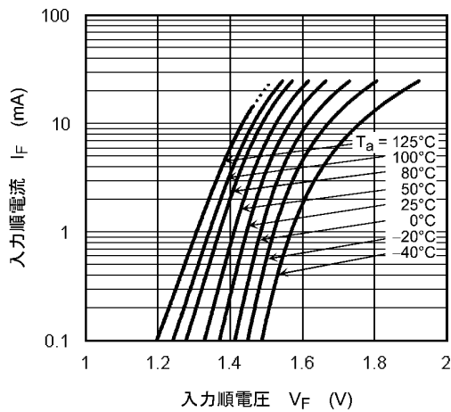
図 12.2.1 I_F - V_F
