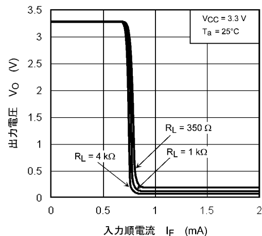
図 12.2.6 V_O - I_F
