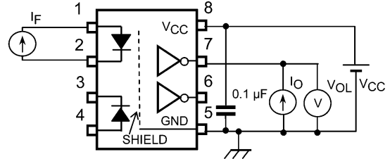
図 12.1.2 VOL測定回路
