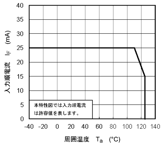
図 12.2.2 I_F - T_a
