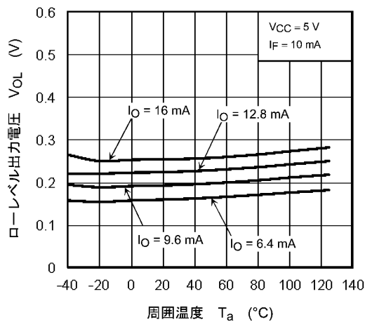
図 12.2.3 V_{OL} - T_a
