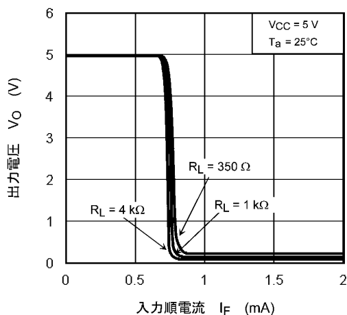
図 12.2.5 V_O - I_F
