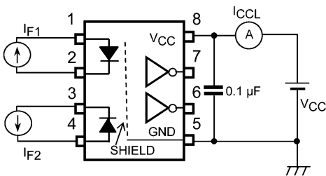
図 12.1.3 ICCL測定回路
