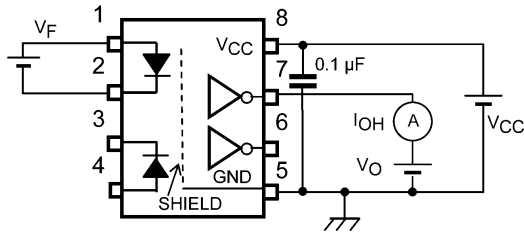
図 12.1.1 IOH測定回路
