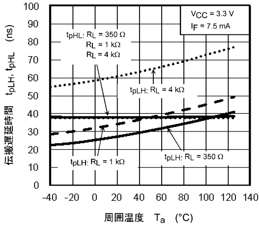
図 12.2.13 t_{pLH} / t_{pHL} - T_a
