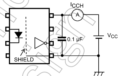
図 12.1.4 I CCH 測定回路
