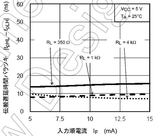
図 12.2.16 |t_{pHL} - t_{pLH}| - I_F
