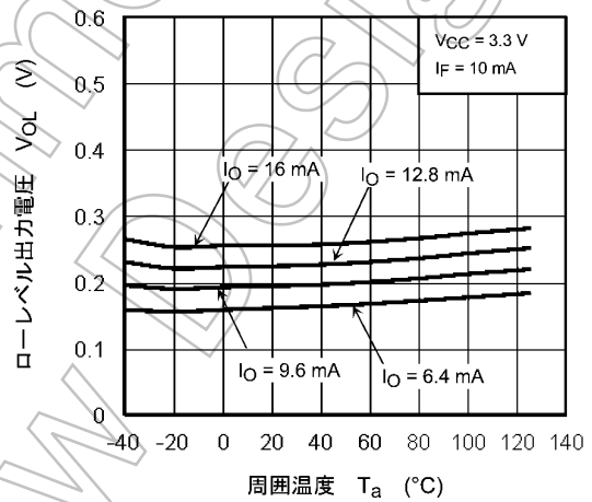
図 12.2.4 V_{OL} - T_a
