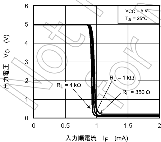
図 12.2.5 V_O - I_F
