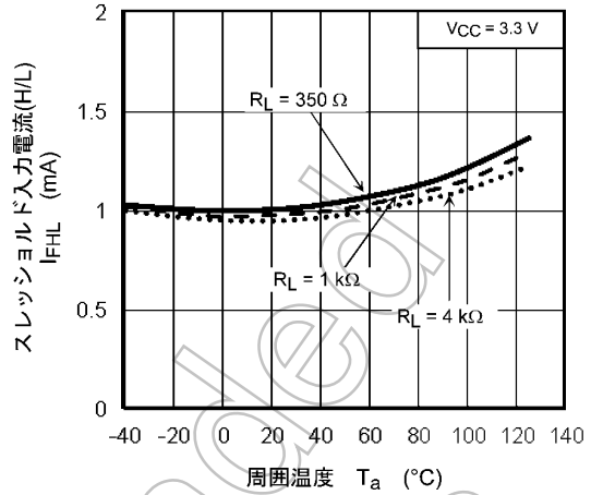
図 12.2.8 I_{FHL} - T_a
