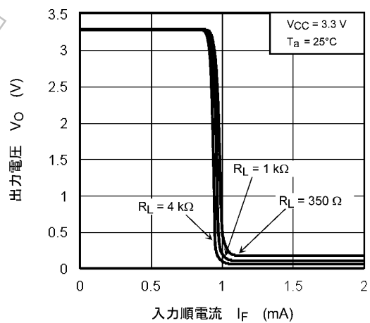
図 12.2.6 V_O - I_F
