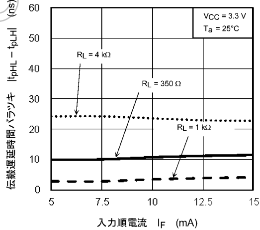
図 12.2.18 |t_{pHL} - t_{pLH}| - I_F
