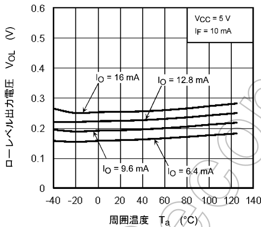
図 12.2.3 V_{OL} - T_a
