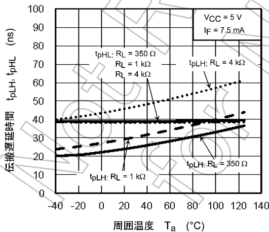
図 12.2.11 t_{pLH} / t_{pHL} - T_a
