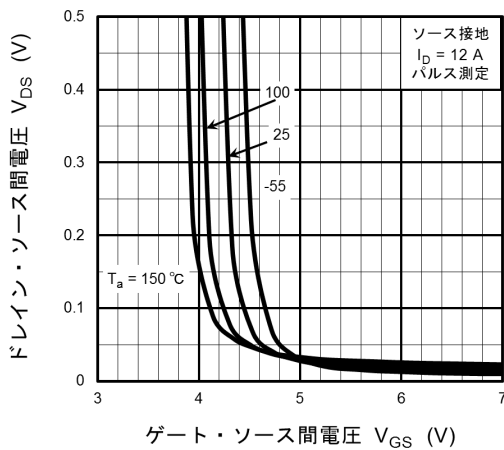
図 8.5 V_{DS} - V_{GS}
