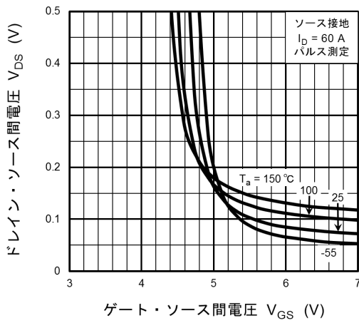
図 8.3 V_{DS} - V_{GS}
