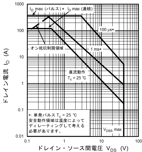
図 8.20 安全動作領域 (最大値 (保証値))
