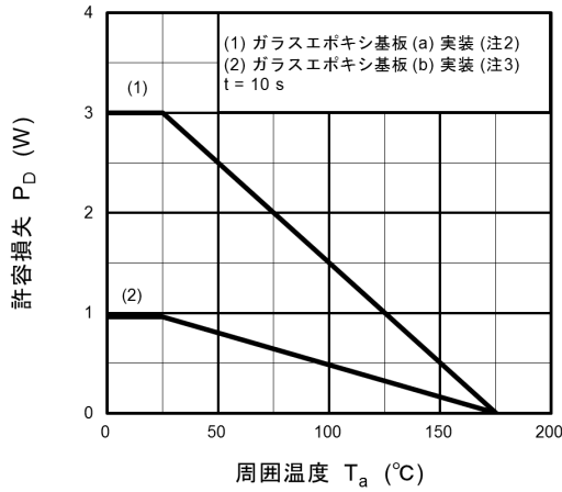
図 8.18 P_D - T_a (最大値 (保証値))
