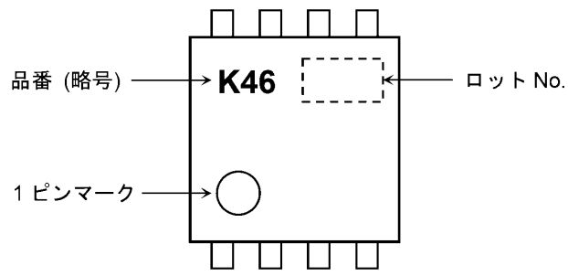
図 7.1 現品表示
