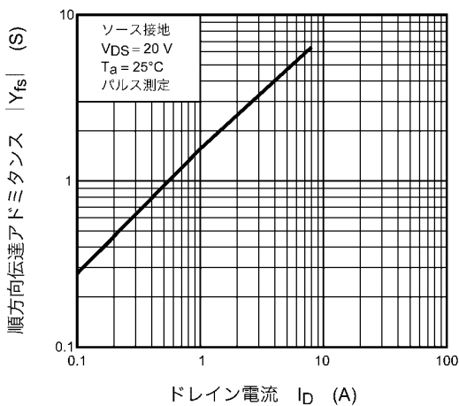
図 8.5 |Y_{fs}| - I_D
