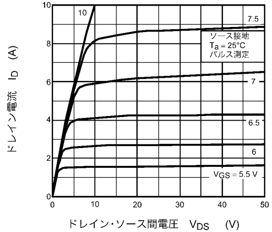
図 8.2 I_D - V_{DS}
