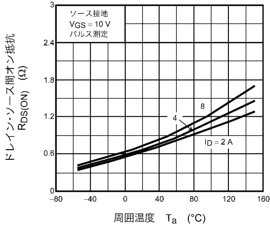
図 8.7 R_{DS(ON)} - T_a
