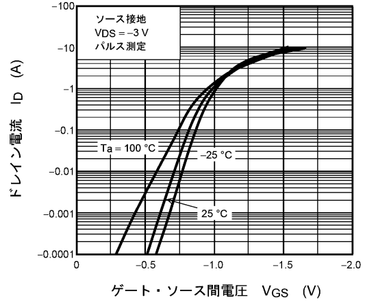
図 7.2 I_D - V_{GS}
