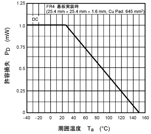
図 8.14 P_D - T_a
