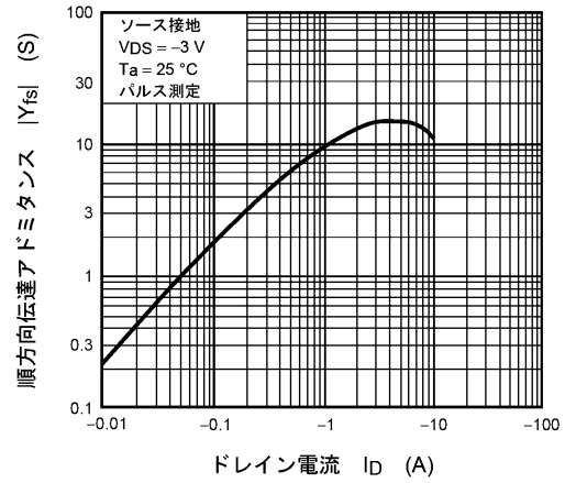
図 7.8 |Y_{fs}| - I_D
