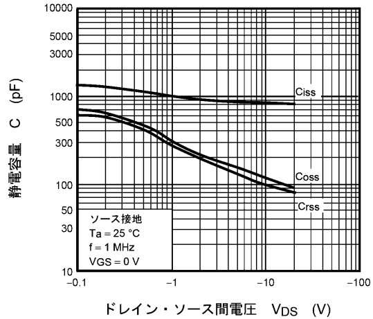
図 8.10 C - V_{DS}
