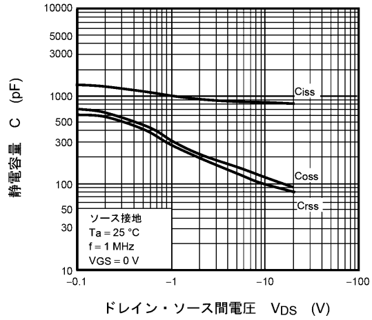
図 7.10 C - V_{DS}
