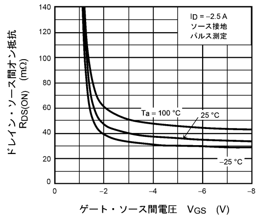
図 7.4 R_{DS(ON)} - V_{GS}
