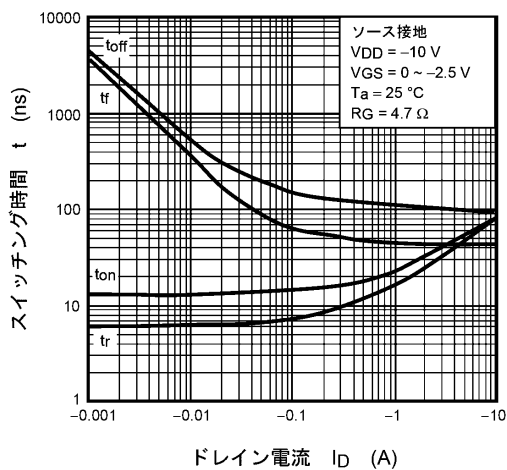
図 7.11 t - I_D
