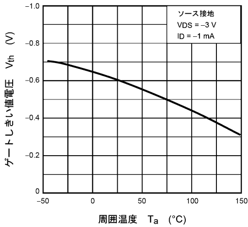
図 7.7 V_{th} - T_a
