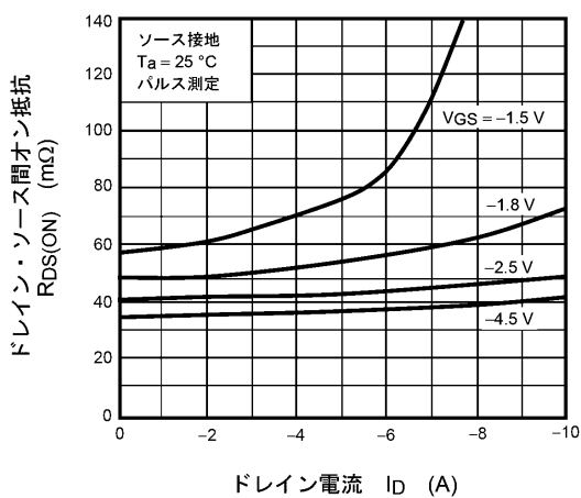
図 7.5 R_{DS(ON)} - I_D
