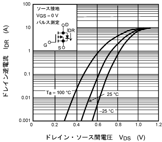
図 8.9 I_{DR} - V_{DS}
