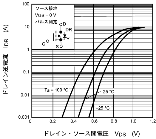
図 7.9 I_{DR} - V_{DS}
