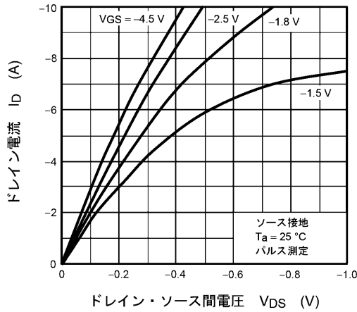
図 7.1 I_D - V_{DS}
