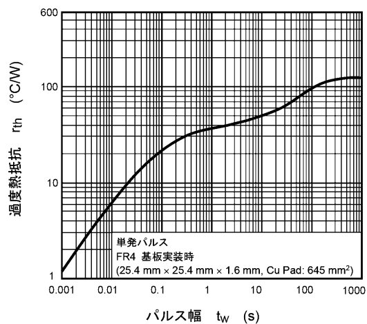
図 7.13 r_{th} - t_w
