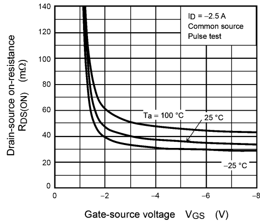
Fig. 7.4 R_{DS(ON)} - V_{GS}
