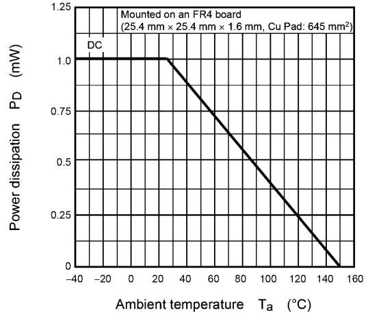
Fig. 7.14 P_D - T_a
