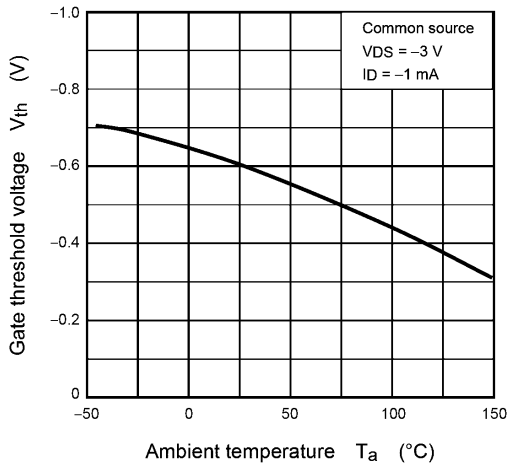
Fig. 7.7 V_{th} - T_a
