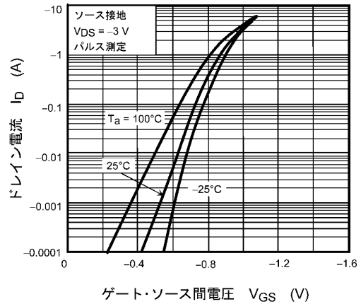
図 7.2 I_D - V_{GS}
