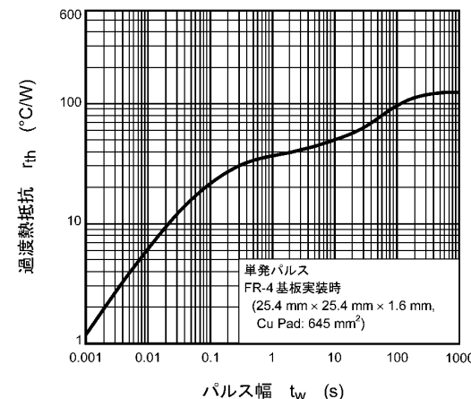
図 7.12 r_{th} - t_w
