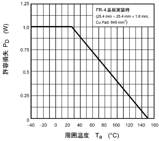
図 7.13 P_D - T_a
