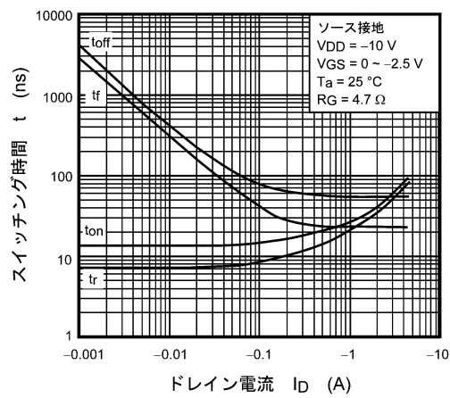
図 8.10 t - ID
