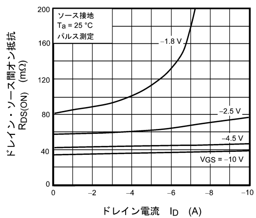
図 8.4 R_{DS(ON)} - I_D
