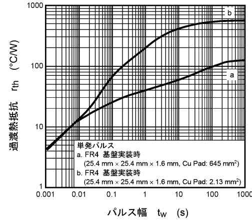
図 8.12 rth - tw
