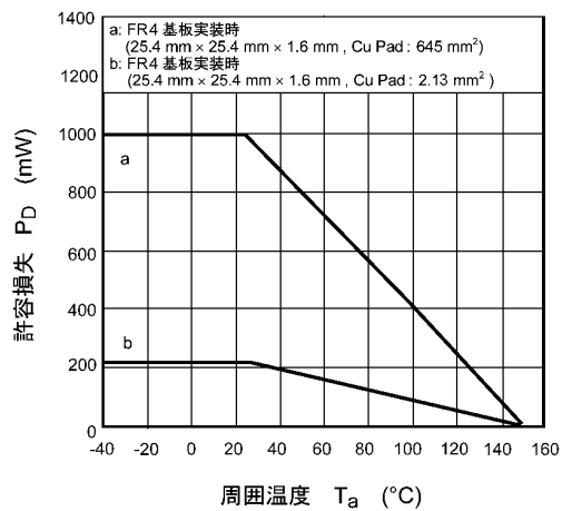
図 8.13 P_D - T_a
