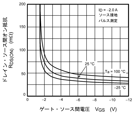
図 8.3 R_{DS(ON)} - V_{GS}
