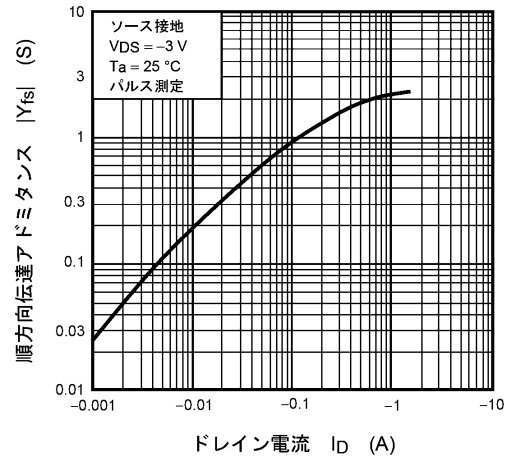
図 7.8 |Y_{fs}| - I_D
