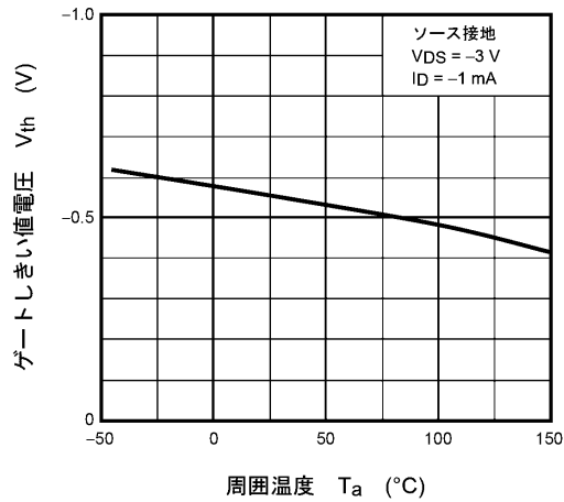
図 7.7 V_{th} - T_a
