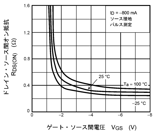
図 7.4 R_{DS(ON)} - V_{GS}
