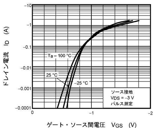
図 7.2 I_D - V_{GS}
