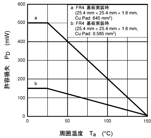
図 7.14 P_D - T_a
