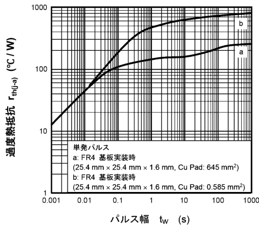
図 7.13 r_{th(j-a)} - t_w
