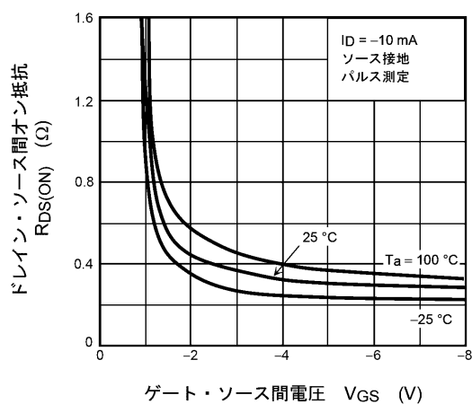
図 7.3 R_{DS(ON)} - V_{GS}
