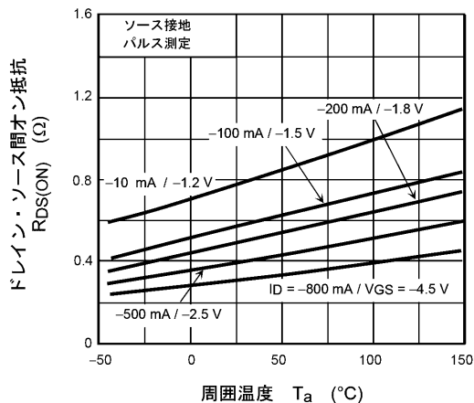
図 7.6 R_{DS(ON)} - T_a
