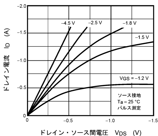
図 7.1 I_D - V_{DS}
