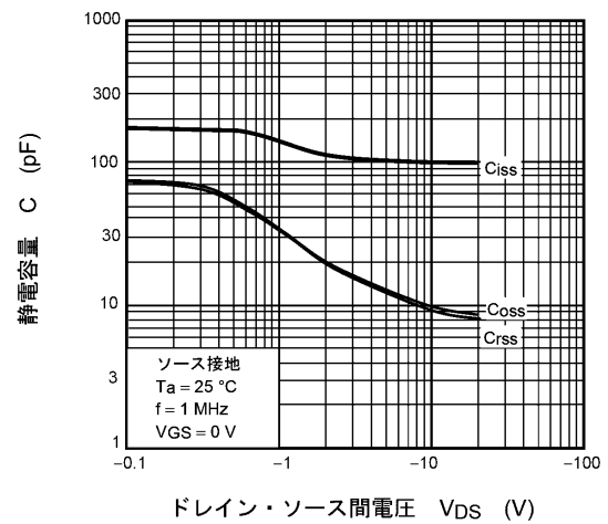
図 7.10 C - V_{DS}
