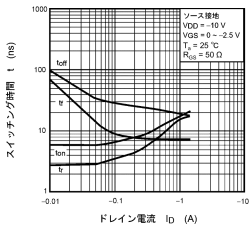
図 7.11 t - I_D
