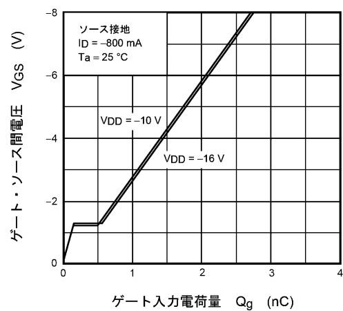
図 7.12 ダイナミック入力特性
