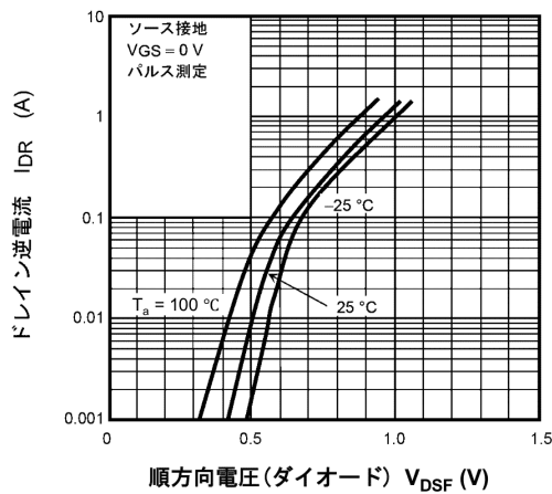
図 7.9 I_{DR} - V_{DSF}
