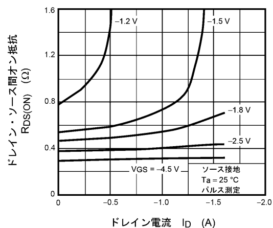
図 7.5 R_{DS(ON)} - I_D
