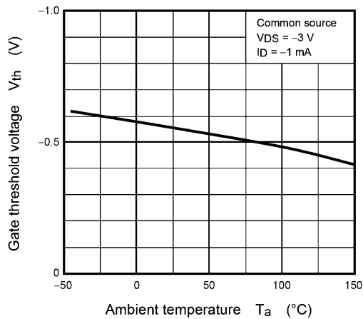
Fig. 7.7 V_{th} - T_a
