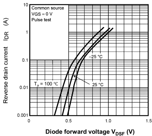
Fig. 7.9 I_{DR} - V_{DSF}
