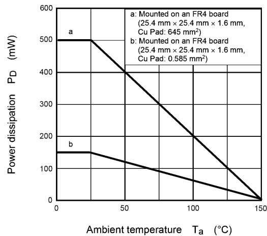
Fig. 7.14 P_D - T_a
