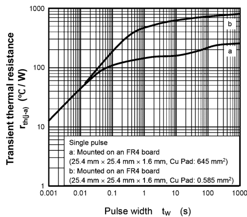
Fig. 7.13 r_{th(j-a)} - t_w
