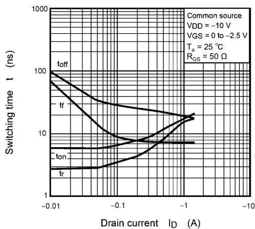
Fig. 7.11 t - I_D
