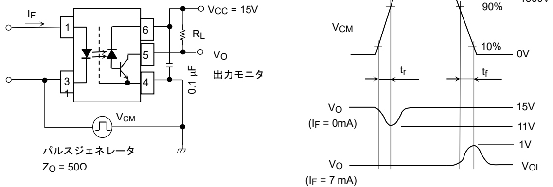
図2 コモンモード過渡耐性測定回路、波形
