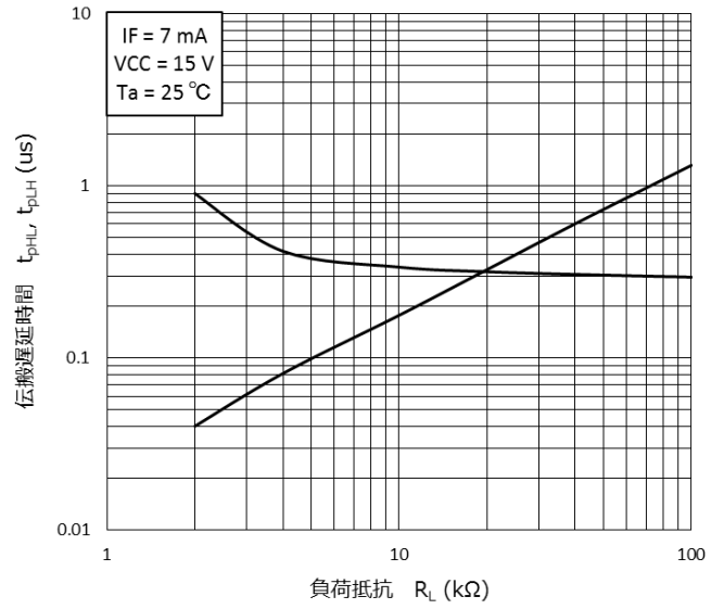
t_{pLH} , t_{pHL} - R_L
