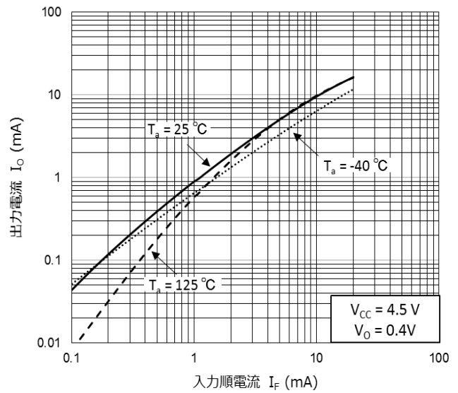
I_O - I_F
