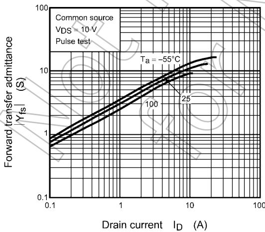
Fig. 8.5 |Y_{fs}| - I_D
