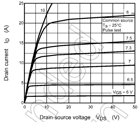
Fig. 8.2 I_D - V_{DS}
