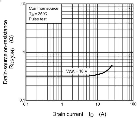
Fig. 8.6 R_{DS(ON)} - I_D
