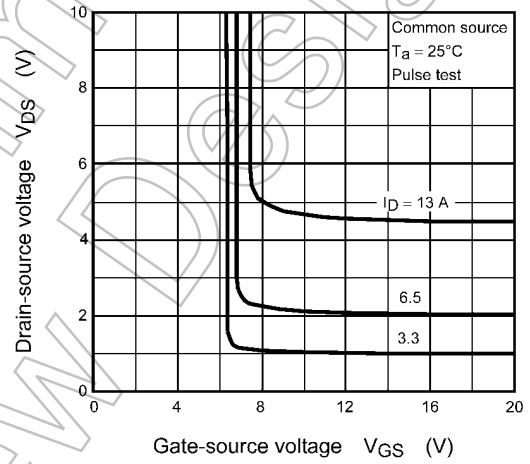
Fig. 8.4 V_{DS} - V_{GS}
