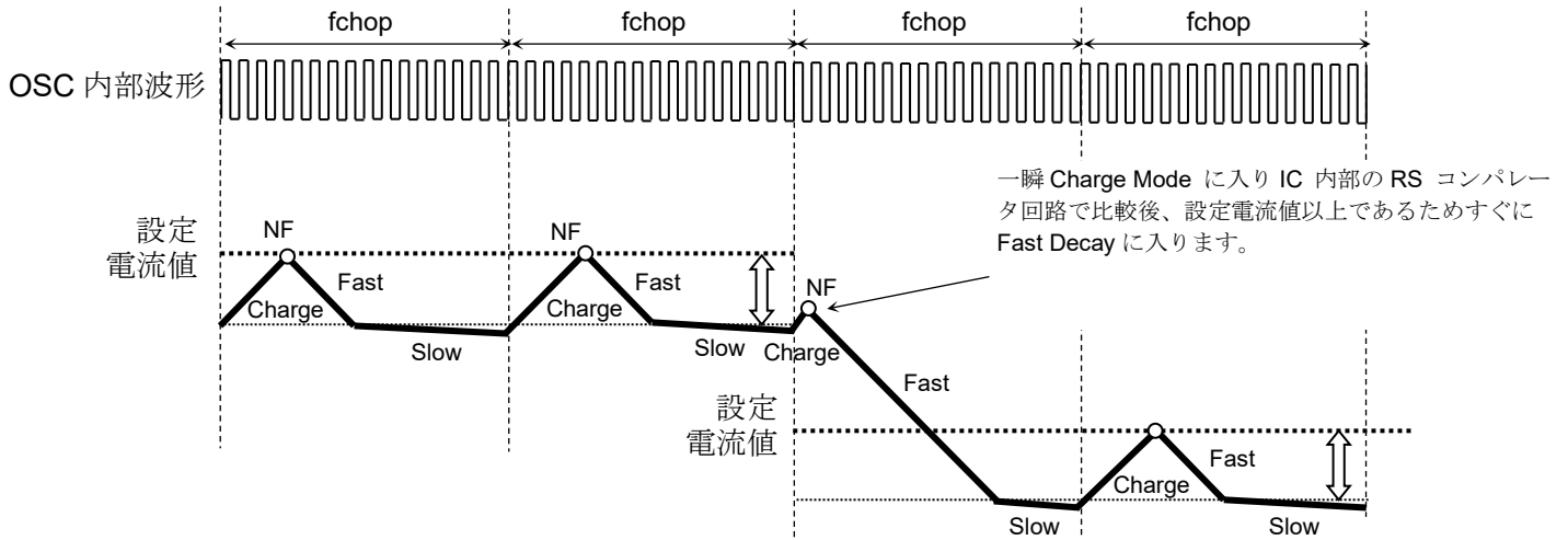
図 8.18 設定電流値が減少方向の場合
