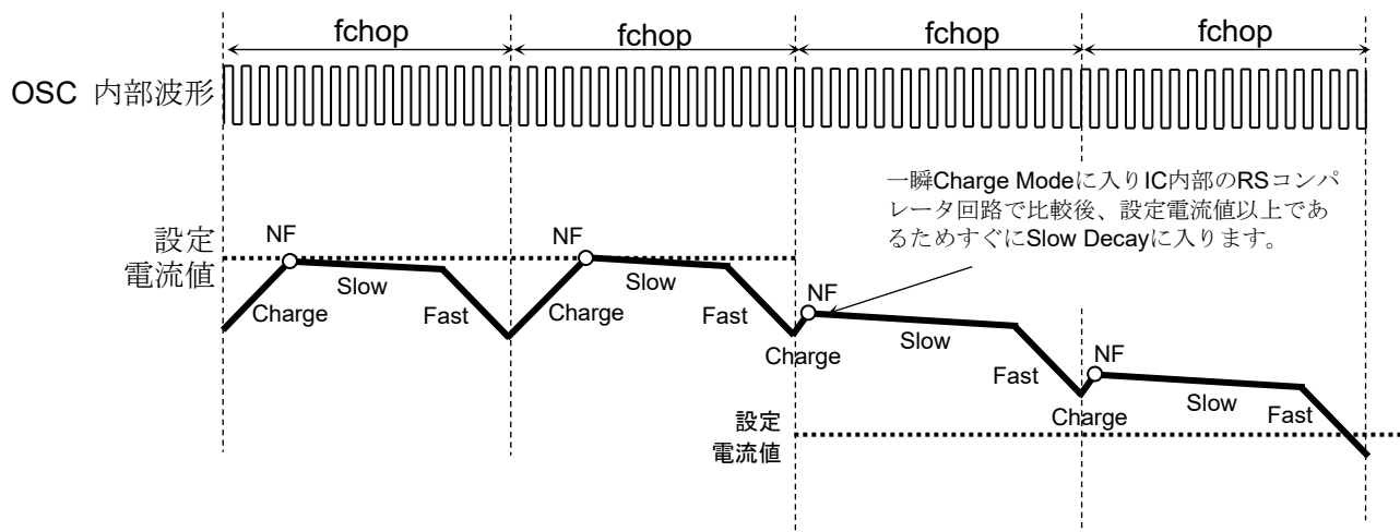
図 8.13 設定電流値が減少方向の場合
