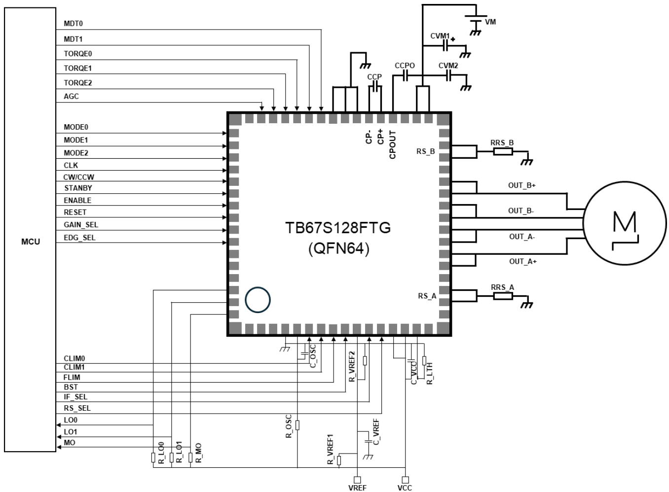
図 14.1 応用回路例
