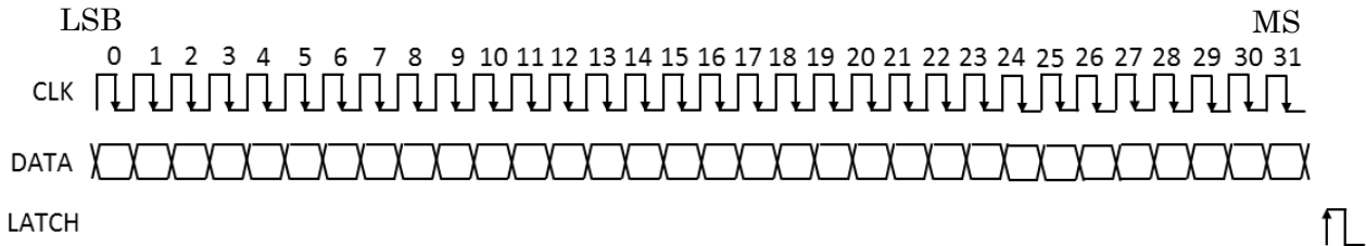
図 9.1 LATCH 信号のタイミング
