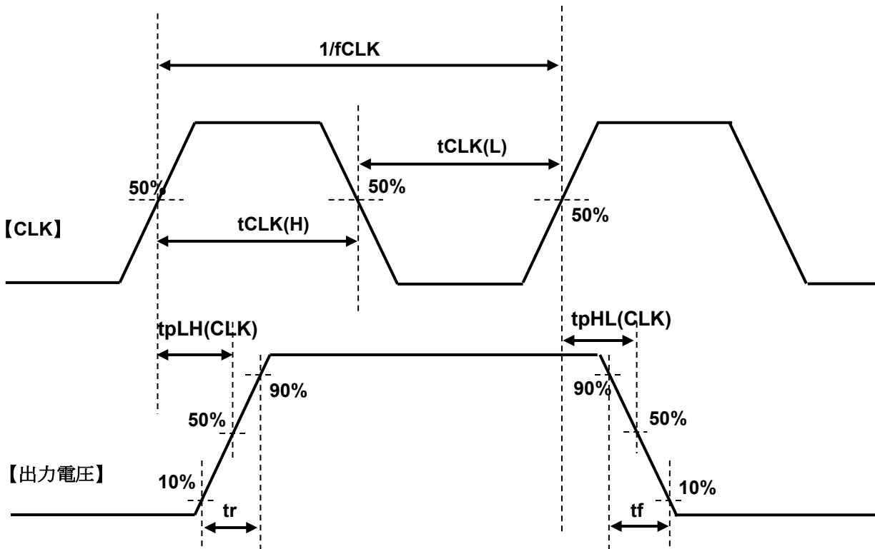
図 13.1 TB67S128FTG(CLK と出力の関係)
