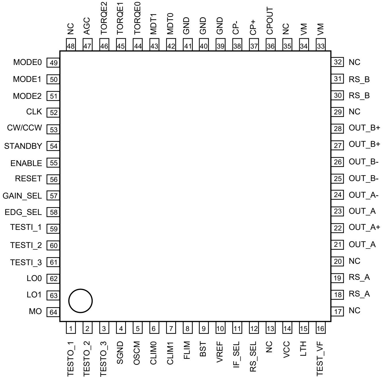
図 3.1 端子配置図
