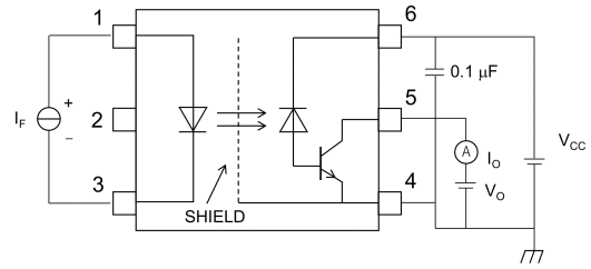
Fig. 13.1.4 IO Test Circuit
