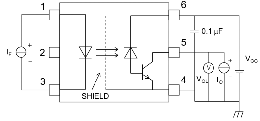
Fig. 13.1.2 VOL Test Circuit
