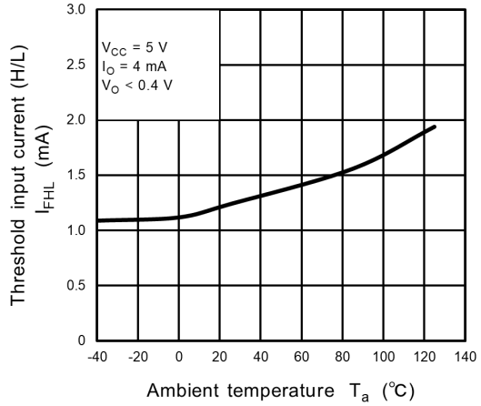
Fig. 14.2.8 I_{FHL} - T_a
