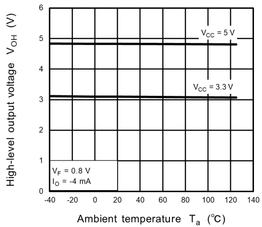
Fig. 14.2.4 V_{OH} - T_a
