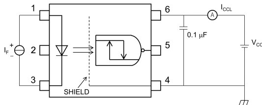
Fig. 14.1.3 I_{CCL} Test Circuit
