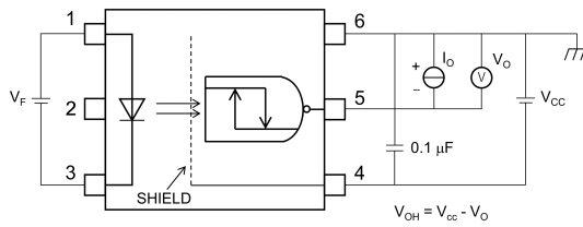
Fig. 14.1.1 V_{OH} Test Circuit
