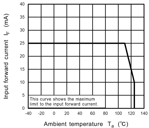
Fig. 14.2.2 I_F - T_a
