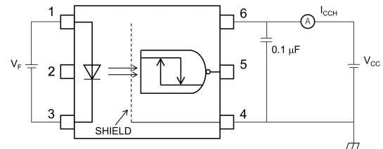
Fig. 14.1.4 I_{CCH} Test Circuit
