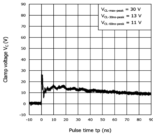
図 6.1.1 +8 kV
