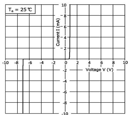
図 9.1 I - V
