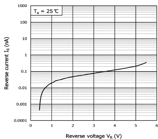
図 9.2 I_R - V_R
