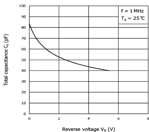
図 9.3 C_t - V_R
