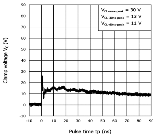
図 6.1.1 +8 kV
