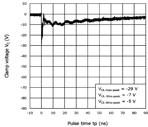
図 6.1.2 -8 kV
