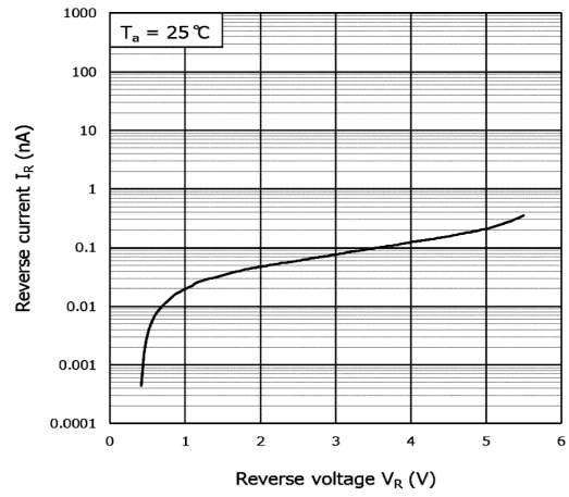
図 9.2 I_R - V_R
