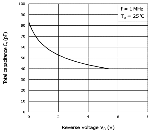
図 9.3 C_t - V_R
