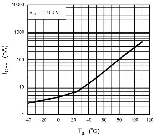
図 12.9 I_{OFF} - T_a
