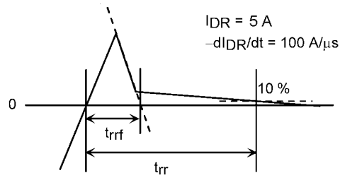
図 6.4.1 逆回復時間
