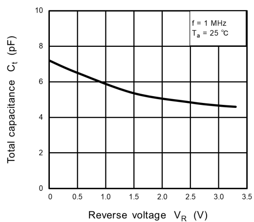
Fig. 9.2 C_t - V_R
