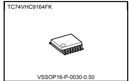
質量 VSSOP16-P-0030-0.50 : 0.02 g (標準)
