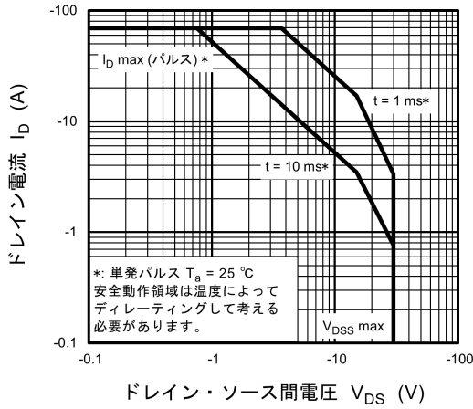
図 8.14 安全動作領域 (最大値 (保証値))
