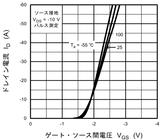
図 8.3 I_D - V_{GS}
