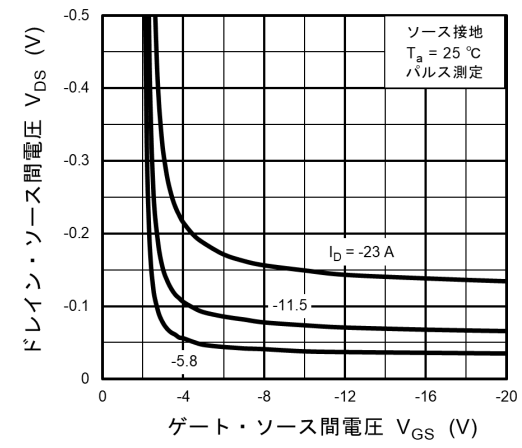
図 8.4 V_{DS} - V_{GS}
