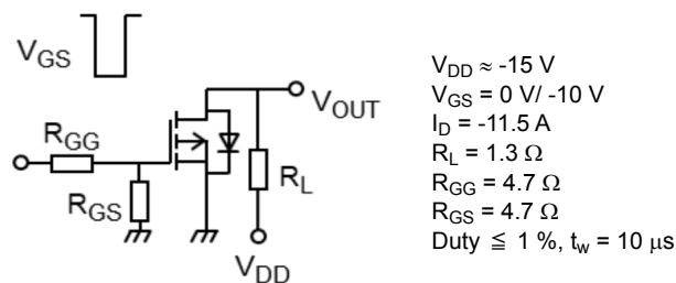
図 6.2.1 スイッチング時間の測定回路図
