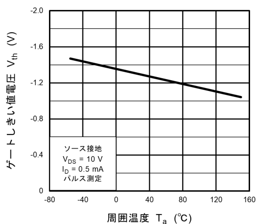
図 8.9 V_{th} - T_a
