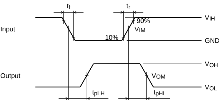
図 2 t_{pLH} , t_{pHL}
