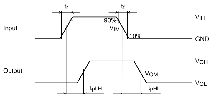
図 2 t_{pLH} , t_{pHL}
