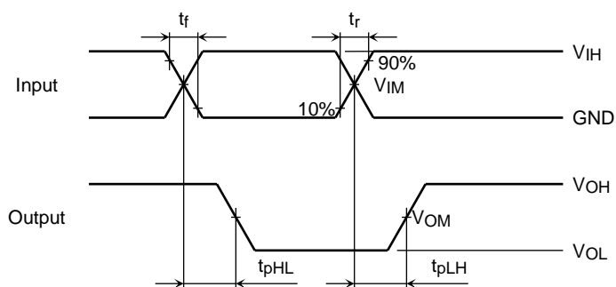
図 2 t_{pLH} , t_{pHL}
