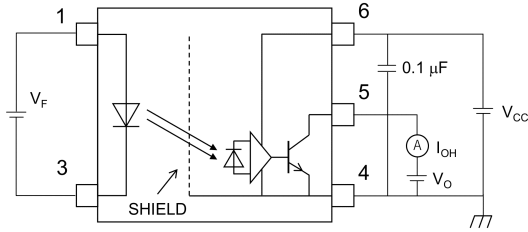
図 12.1.1 I OH 測定回路
