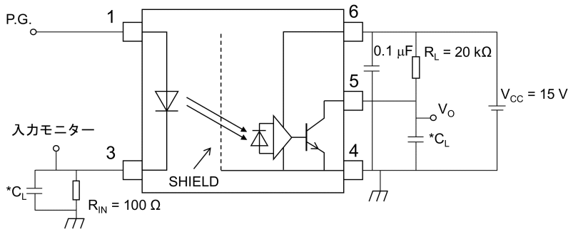
図 12.1.6 伝搬遅延時間測定回路, 波形
