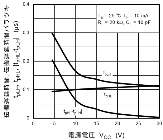
図 12.2.12 t_{pLH}, t_{pHL}, |t_{pHL} - t_{pLH}| - V_{CC}
