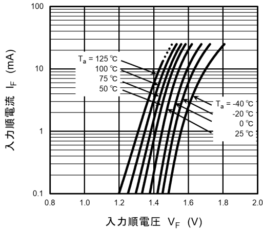
図 12.2.1 I_F - V_F
