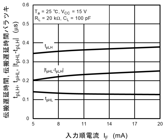
図 12.2.15 t_{pLH} , t_{pHL} , |t_{pHL} - t_{pLH}| - I_F
