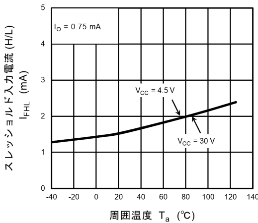
図 12.2.3 I_{FHL} - T_a
