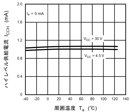
図 12.2.6 I_{CCH} - T_a
