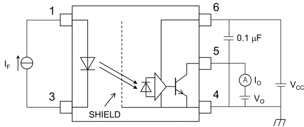
図 12.1.5 I O 測定回路
