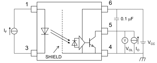
図 12.1.2 V OL 測定回路
