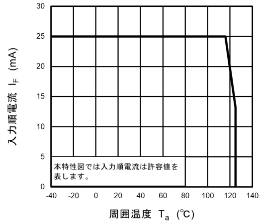
図 12.2.2 I_F - T_a
