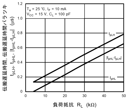
図 12.2.17 t_{pLH} , t_{pHL} , |t_{pHL} - t_{pLH}| - R_L
