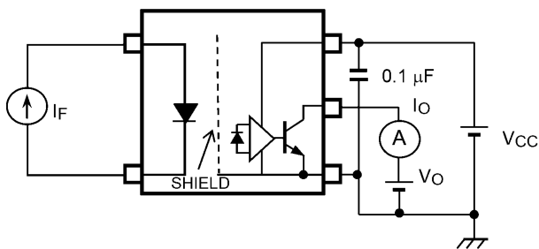
図 12.1.5 I O 測定回路
