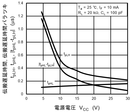
図 12.2.13 t_{pLH} , t_{pHL} , |t_{pHL} - t_{pLH}| - V_{CC}
