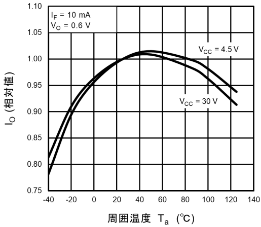
図 12.2.7 I_O - T_a
