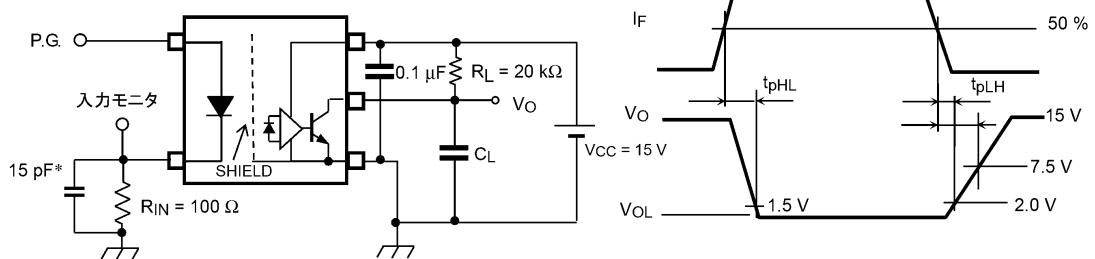
図 12.1.6 伝搬遅延時間測定回路, 波形
