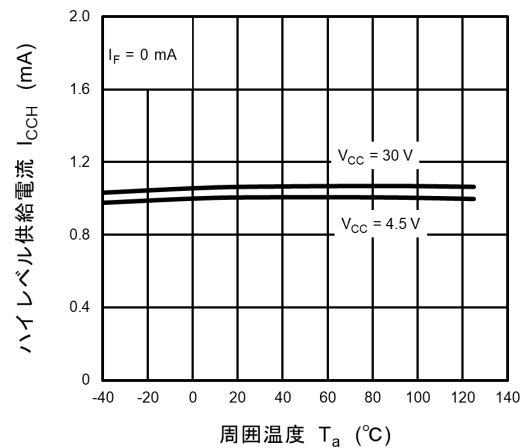
図 12.2.6 I_{CCH} - T_a
