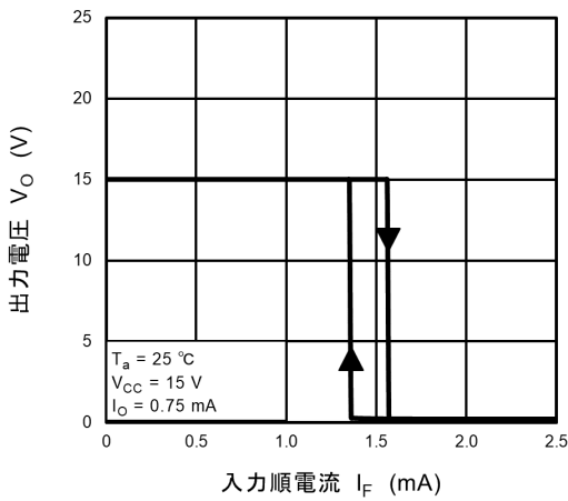
図 12.2.9 V_O - I_F
