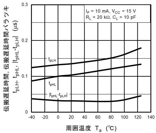
図 12.2.10 t_{pLH}, t_{pHL}, |t_{pHL} - t_{pLH}| - T_a
