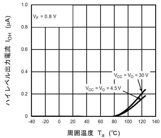
図 12.2.4 I_{OH} - T_a
