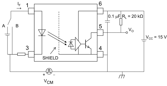
図 12.1.7 コモンモード過渡耐性測定回路, 波形
