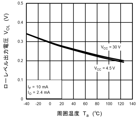
図 12.2.8 V_{OL} - T_a
