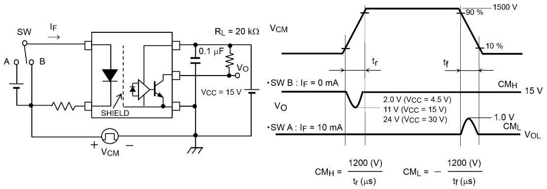
図 12.1.7 コモンモード過渡耐性測定回路, 波形
