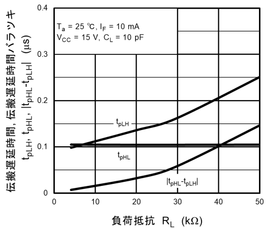
図 12.2.16 t_{pLH} , t_{pHL} , |t_{pHL} - t_{pLH}| - R_L
