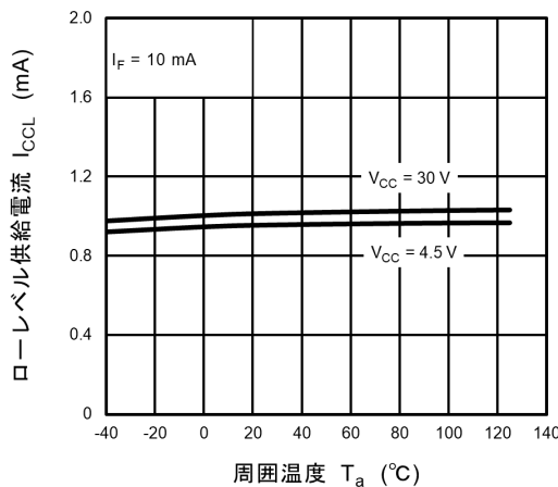
図 12.2.5 I_{CCL} - T_a
