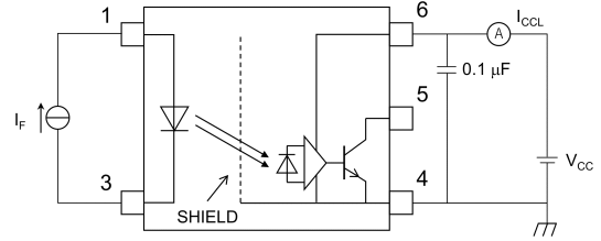
図 12.1.4 I CCL 測定回路
