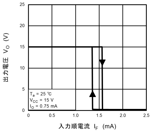
図 12.2.9 V_O - I_F
