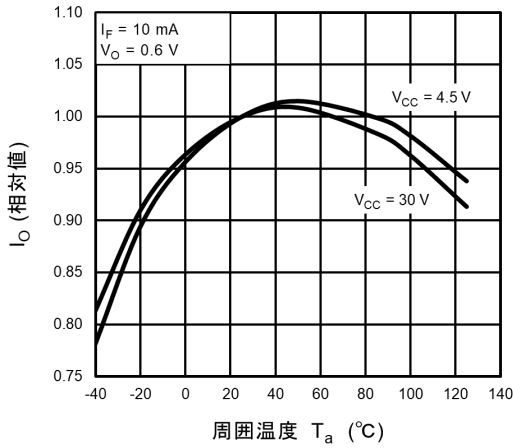
図 12.2.7 I_O - T_a
