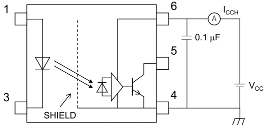
図 12.1.3 I CCH 測定回路
