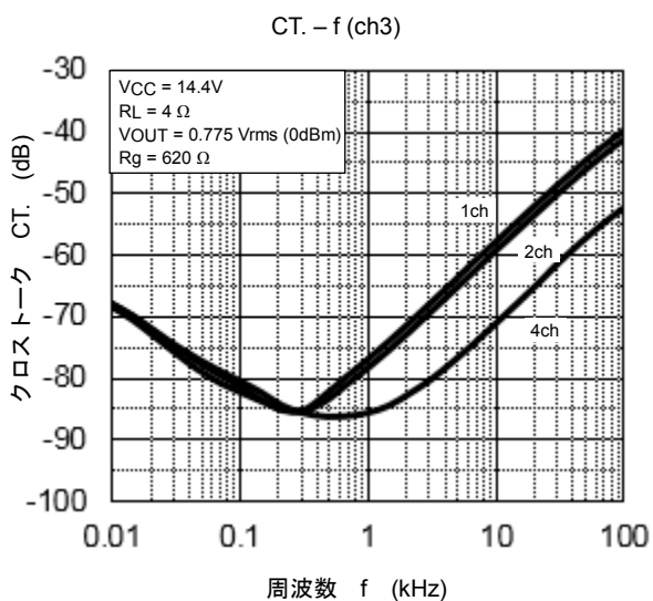
図 18-6 クロストークの周波数特性
