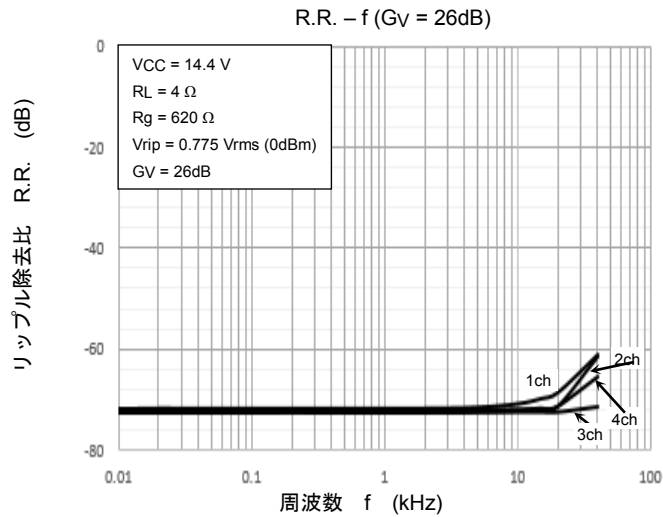
図 18-5 リップル除去比の周波数特性
