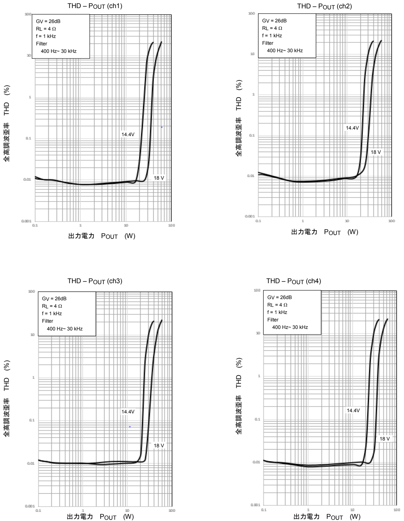
図 18-2 電源電圧による全高調波歪率 (RL = 4 Ω)
