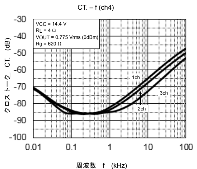
図 18-6 クロストークの周波数特性
