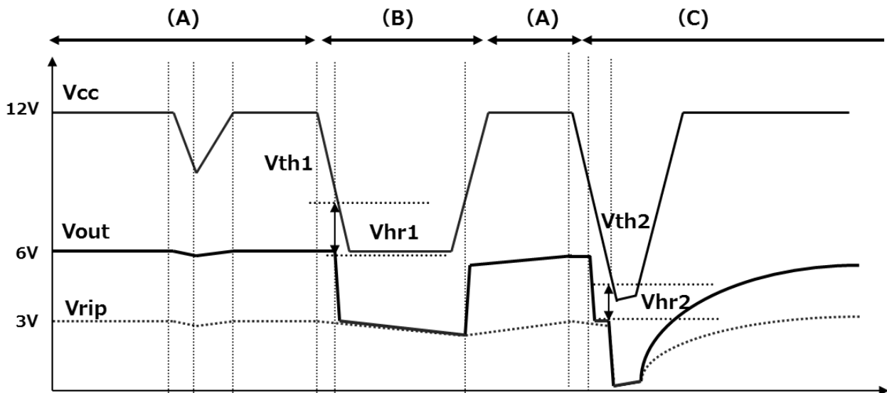
図 12 Vcc 低下時の出力中点電位
