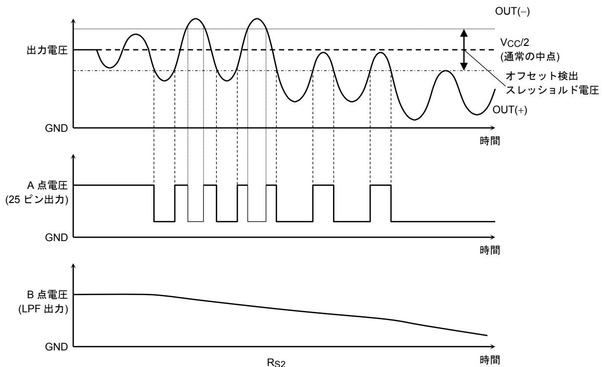
図 7 アンプ出力波形および 25 ピン出力波形
