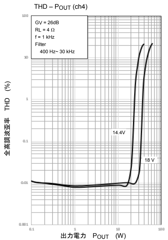
図 18-2 電源電圧による全高調波歪率 (RL = 4 Ω)
