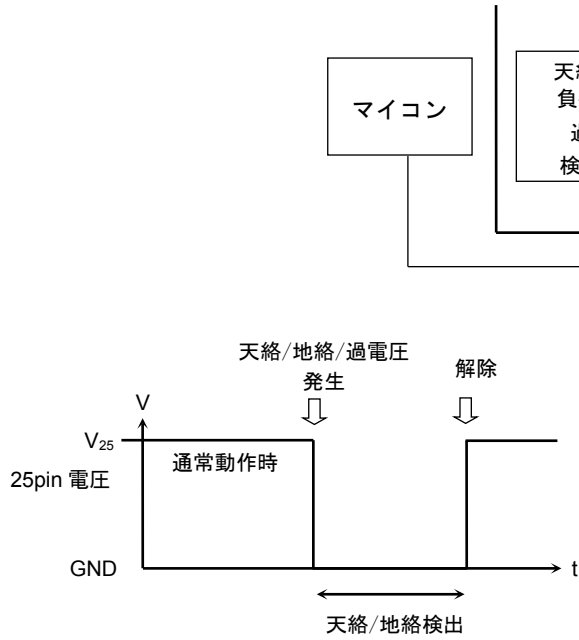
図 8 出力ショート検出時 出力波
