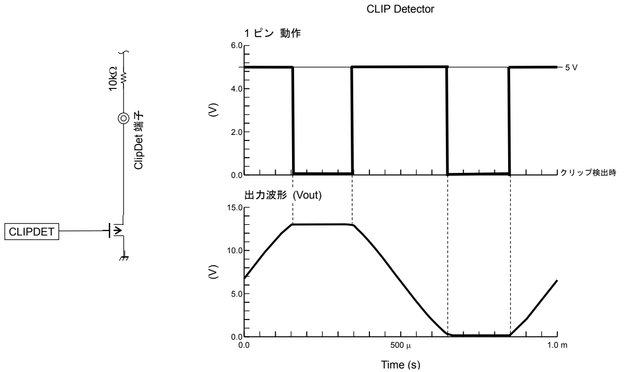
図 10 端子 1 機能オープンドレイン出力
