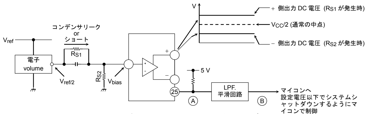
図 6 異常出力オフセット電圧の発生メカニズム
