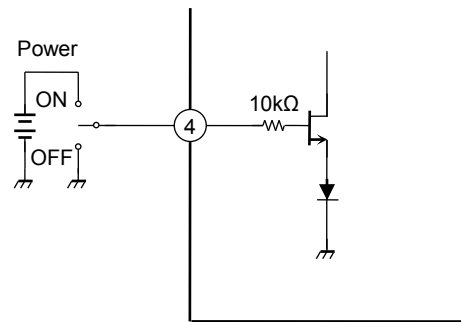
図 1 スタンバイ回路図
