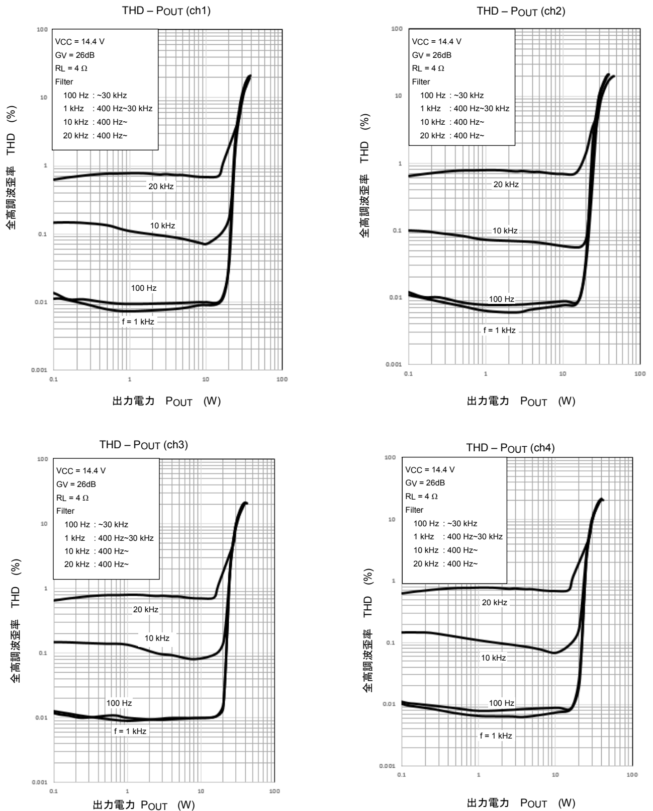
図 18-1 周波数ごとの全高調波歪率 (RL = 4 Ω)
