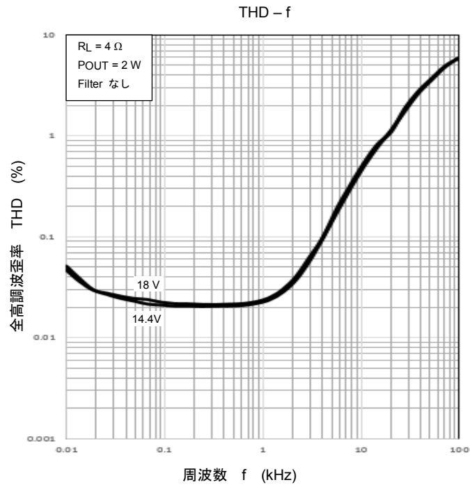
図 188-3 全高調波歪率の周波数特性
