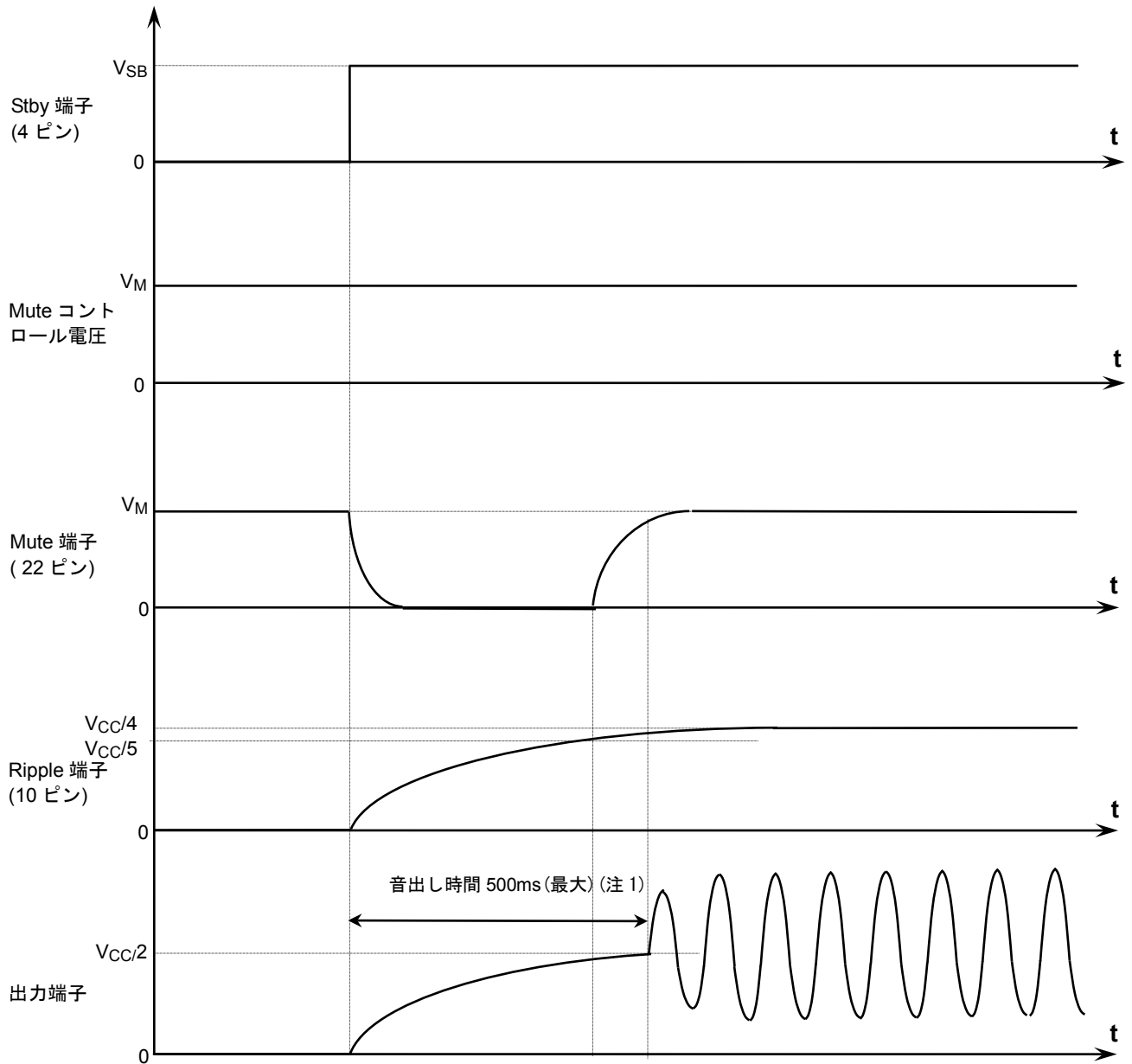
図4 スタンバイ OFF 後のミュート動作シーケンス
