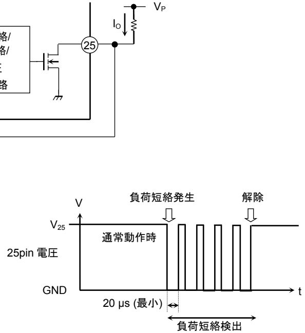
図 9 負荷短絡検出時 出力波形
