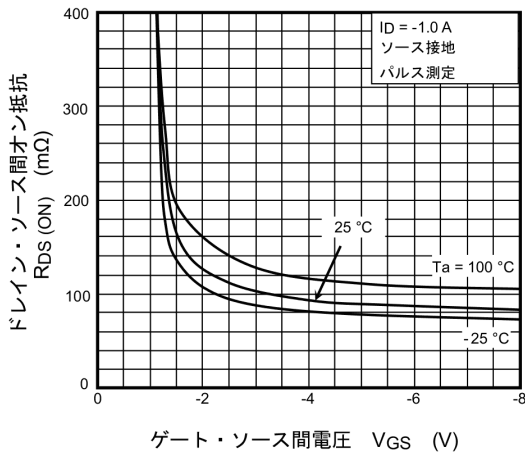
図 7.1.3 R_{DS(ON)} - V_{GS}
