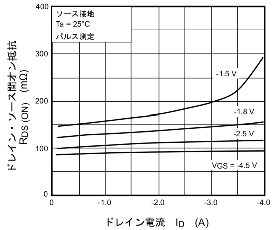
図 7.1.4 R_{DS(ON)} - I_D
