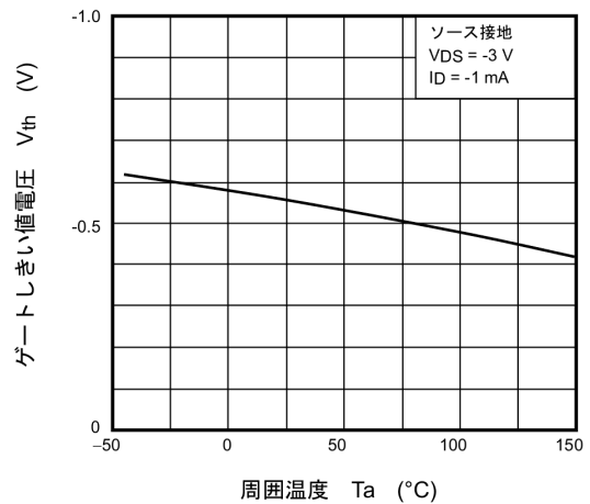
図 7.1.6 V_{th} - T_a
