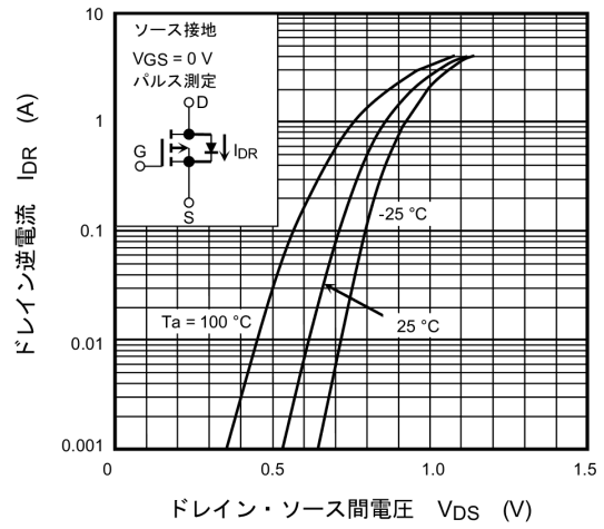
図 7.1.8 I_{DR} - V_{DS}
