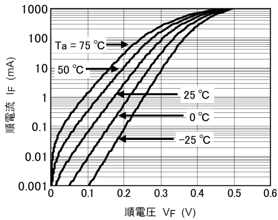
図 7.2.1 I_F - V_F
