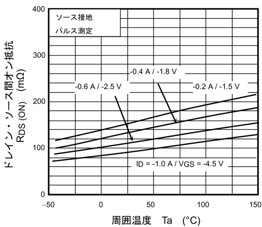
図 7.1.5 R_{DS(ON)} - T_a
