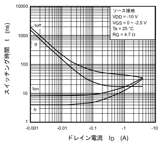
図 7.1.10 t - I_D
