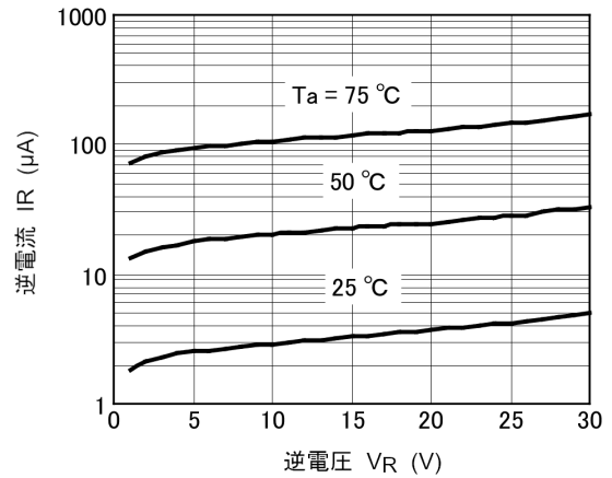
図 7.2.2 I_R - V_R
