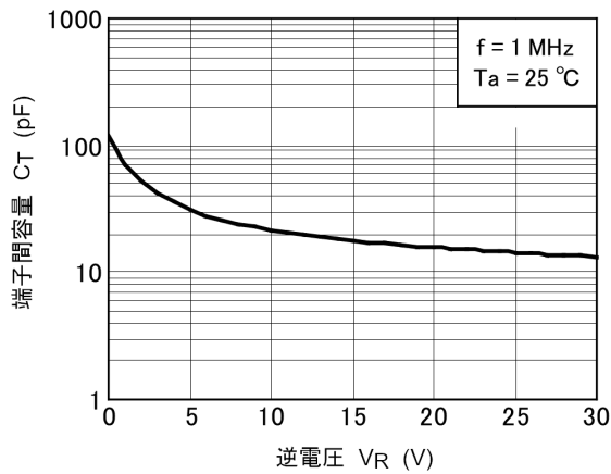
図 7.2.3 C_t - V_R
