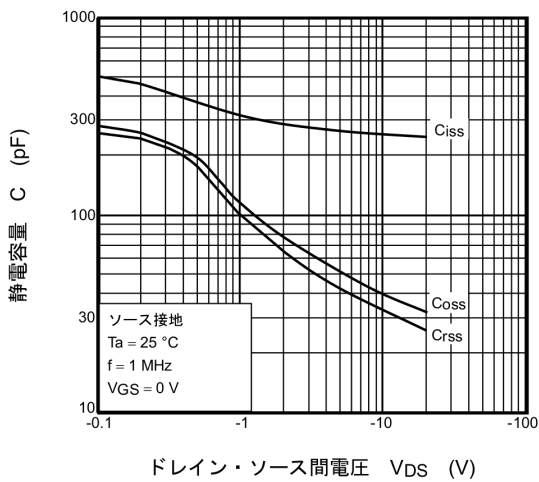
図 7.1.9 C - V_{DS}
