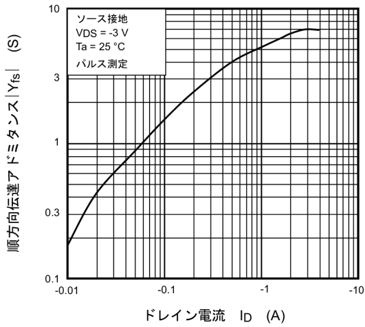
図 7.1.7 |Y_{fs}| - I_D
