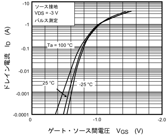
図 7.1.2 I_D - V_{GS}
