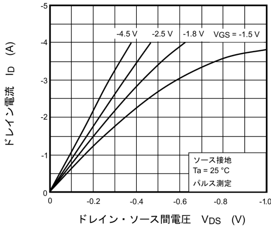
図 7.1.1 I_D - V_{DS}
