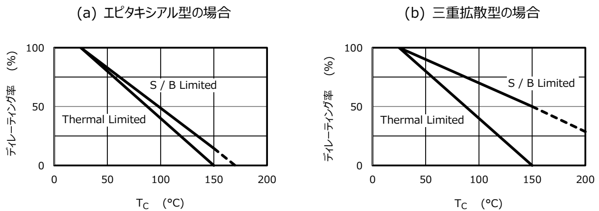
図 1.18 SOA の温度デレージング例
