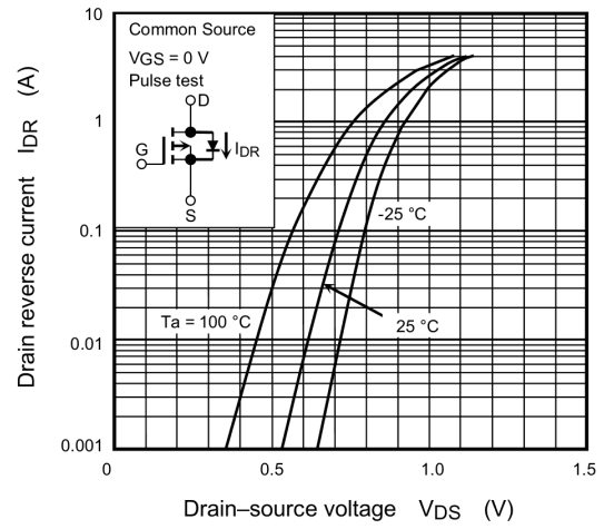
Fig. 7.1.8 I_{DR} - V_{DS}
