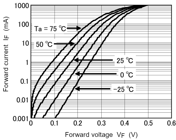
Fig. 7.2.1 I_F - V_F
