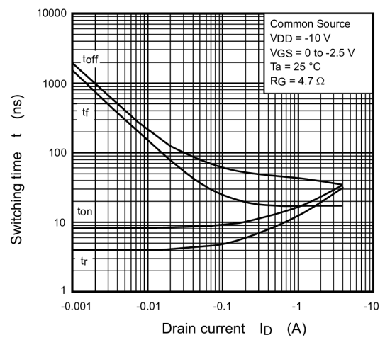
Fig. 7.1.10 t - I_D
