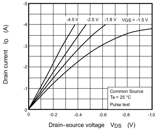
Fig. 7.1.1 I_D - V_{DS}
