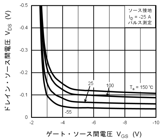
図 8.4 V_{DS} - V_{GS}
