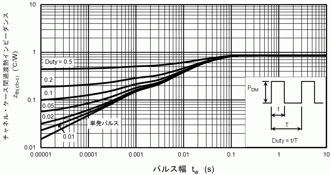
図 8.18 Z_{th(ch-c)} - t_w (最大値(保証値))
