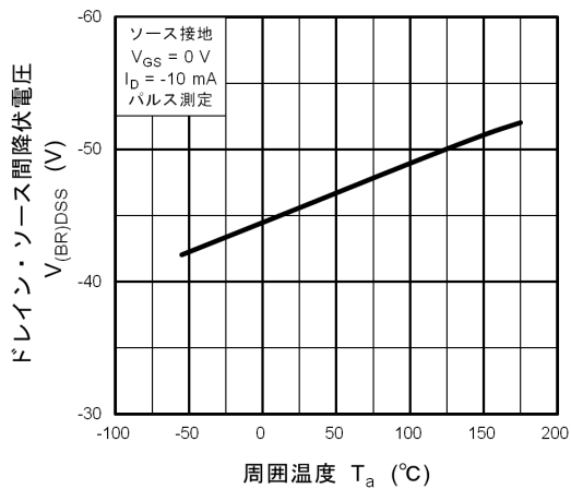
図 8.11 V_{(BR)DSS} - T_a
