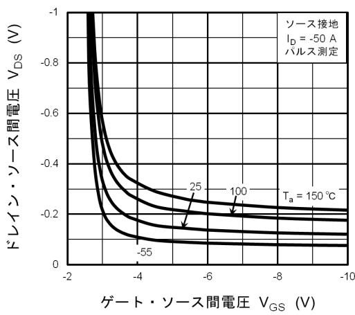
図 8.3 V_{DS} - V_{GS}
