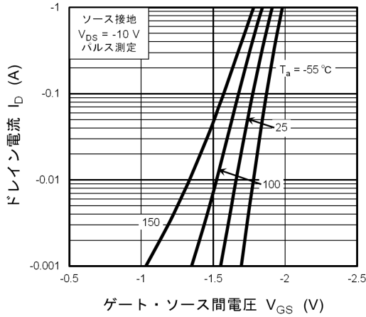
図 8.7 I_D - V_{GS}
