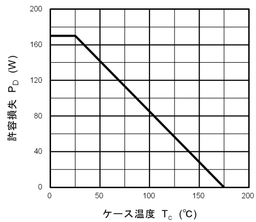
図 8.16 P_D - T_c (最大値(保証値))
