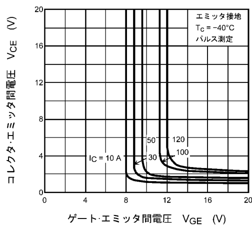
図 8.6 V_{CE} - V_{GE}
