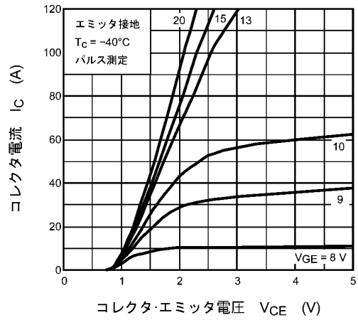
図 8.2 I_C - V_{CE}
