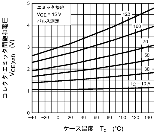
図 8.9 V_{CE(sat)} - T_c
