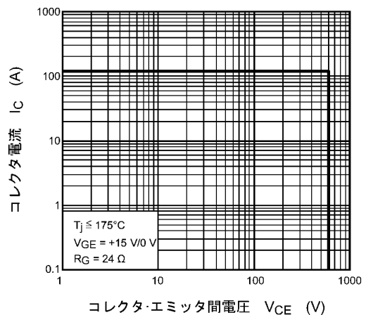
図 8.18 逆バイアス安全動作領域 (最大値 (保証値))
