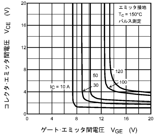
図 8.8 V_{CE} - V_{GE}
