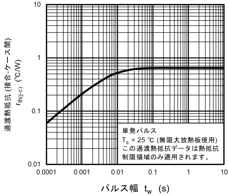
図 8.19 r_{th(j-c)} - t_w (最大值 (保証値))
