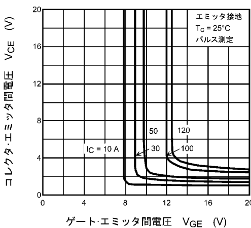
図 8.5 V_{CE} - V_{GE}
