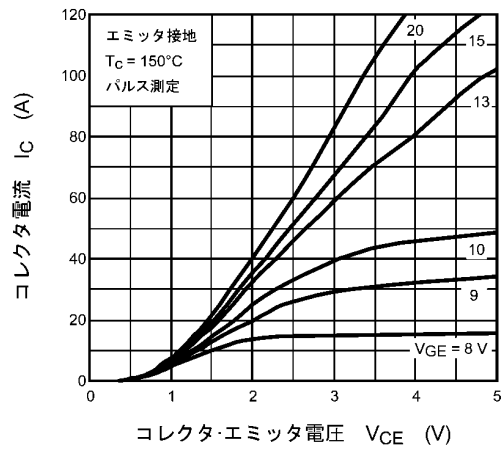
図 8.4 I_C - V_{CE}
