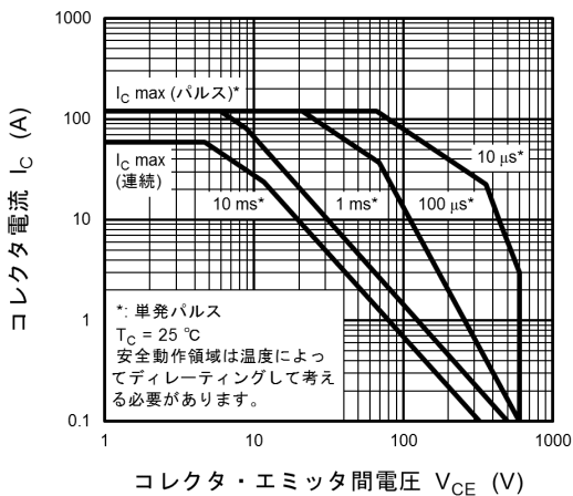
図 8.17 安全動作領域 (最大値 (保証値))
