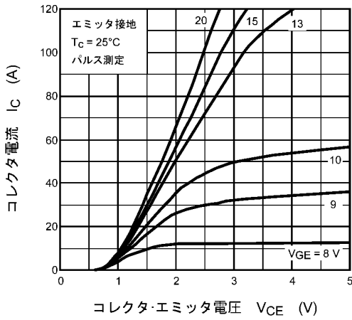
図 8.1 I_C - V_{CE}
