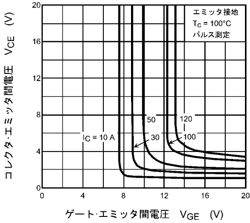
図 8.7 V_{CE} - V_{GE}
