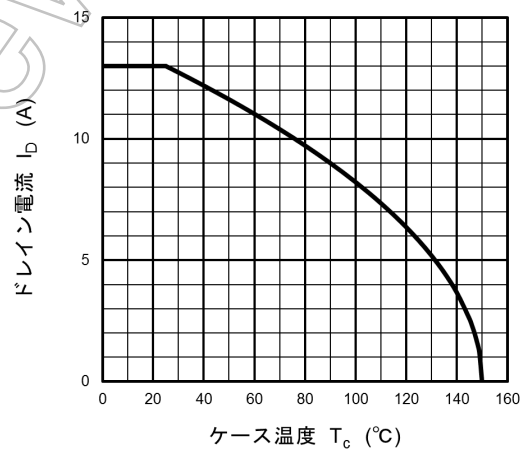
図 8.12 I D - T c (最大値 (保証値))
