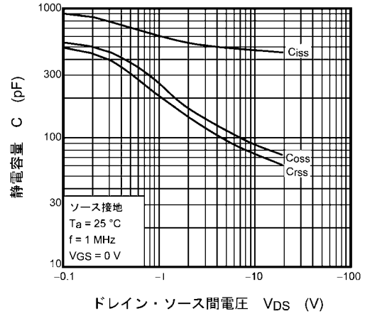
図 7.2.8 C - V_{DS}
