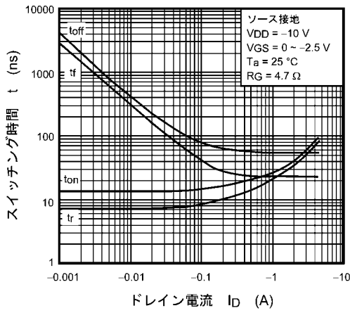
図 7.2.9 t - I_D
