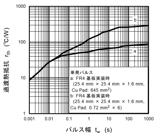
図 7.3.1 r_{th} - t_w
