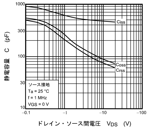
図 8.2.8 C - V DS
