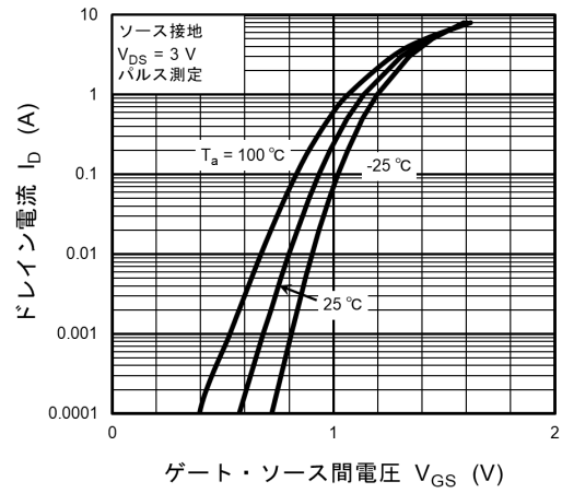
図 7.1.2 I_D - V_{GS}
