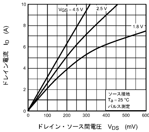
図 8.1.1 I_D - V_{DS}
