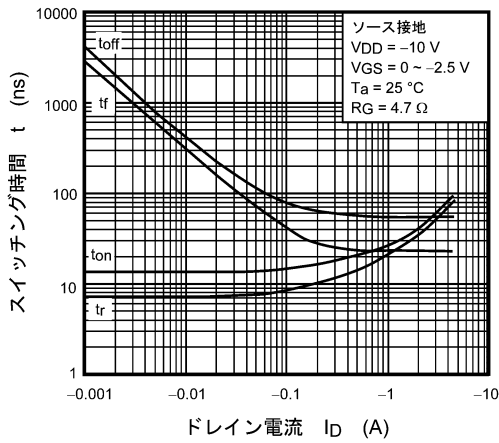
図 8.2.9 t - I D
