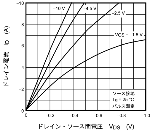
図 7.2.1 I_D - V_{DS}
