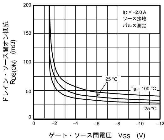
図 8.2.3 R_{DS(ON)} - V_{GS}
