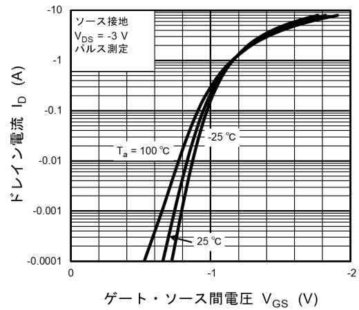
図 8.2.2 I_D - V_{GS}
