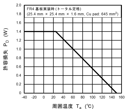
図 7.3.2 P_D - T_a
