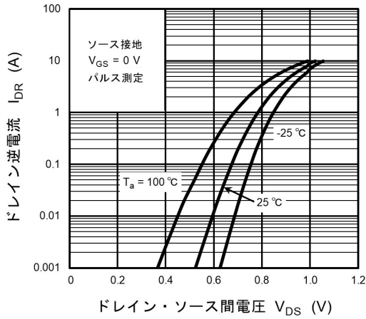
図 8.2.7 I DR - V DS
