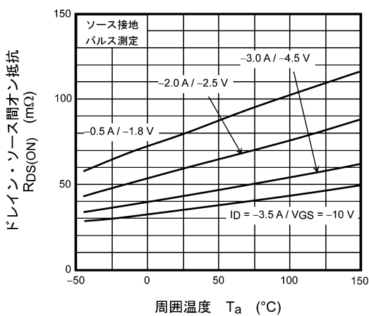
図 8.2.5 R_{DS(ON)} - T_a
