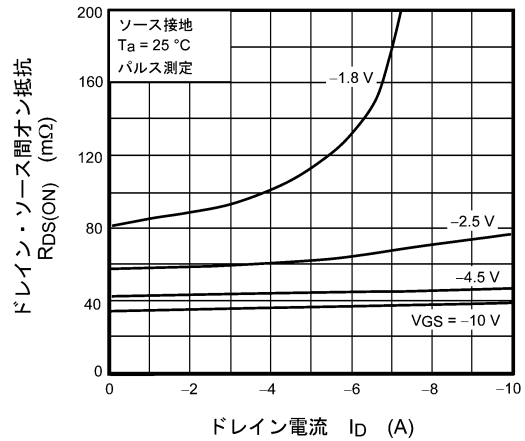
図 7.2.4 R_{DS(ON)} - I_D
