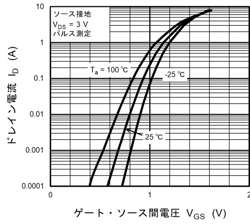
図 8.1.2 I_D - V_{GS}
