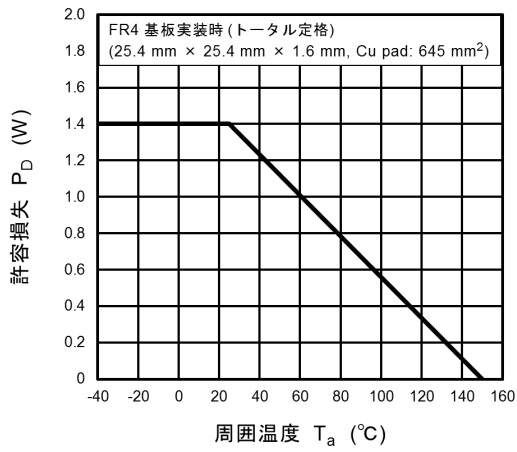
図 8.3.1 P_D - T_a
