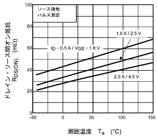
図 8.1.6 R_{DS(ON)} - T_a
