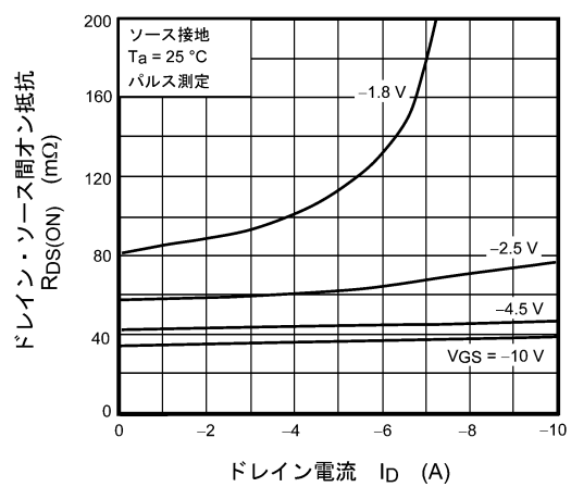
図 8.2.4 R_{DS(ON)} - I_D
