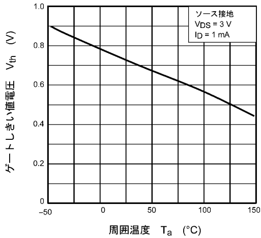
図 8.1.7 V_{th} - T_a
