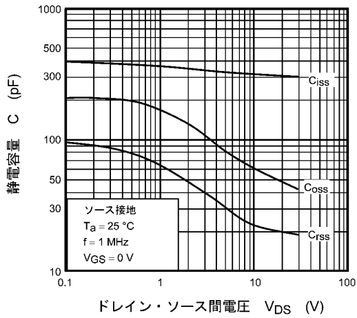
図 8.1.9 C - V_{DS}
