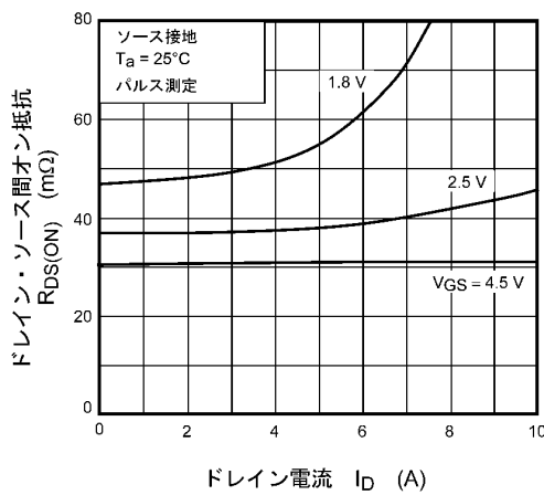
図 8.1.5 R_{DS(ON)} - I_D
