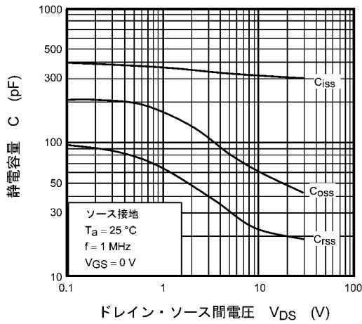
図 7.1.9 C - V_{DS}
