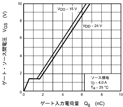
図 8.1.11 ダイナミック入力特性
