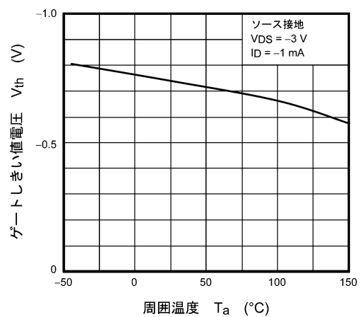
図 8.2.6 V_{th} - T_a
