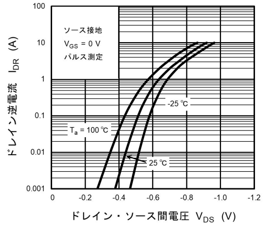
図 8.1.8 I_{DR} - V_{DS}
