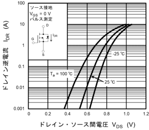
図 7.2.7 I_{DR} - V_{DS}
