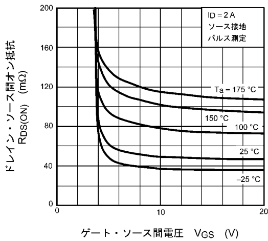
図 7.3 R_{DS(ON)} - V_{GS}
