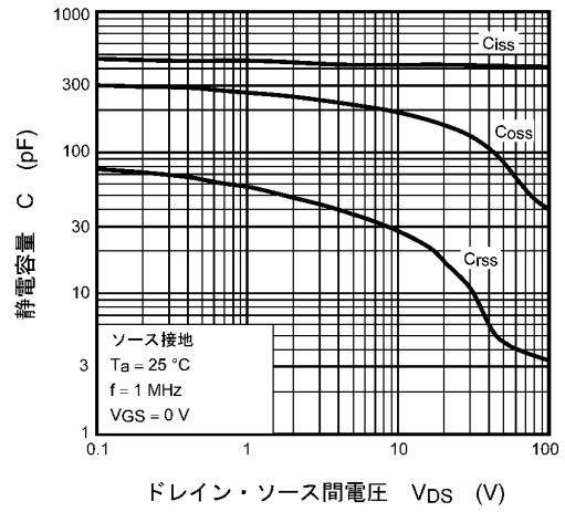
図 7.8 C - Vds
