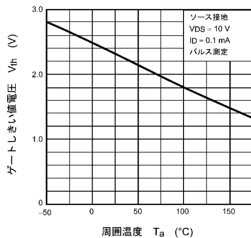
図 7.6 V_{th} - T_a
