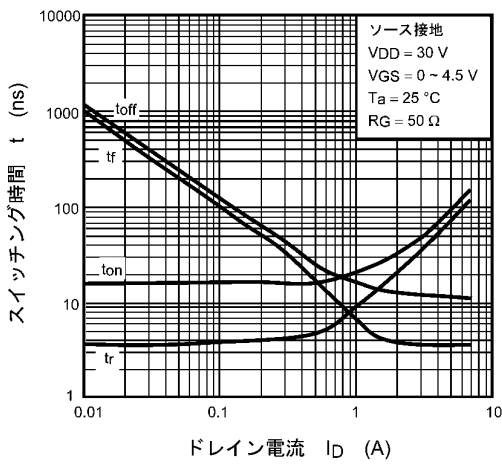
図 7.9 t - Id
