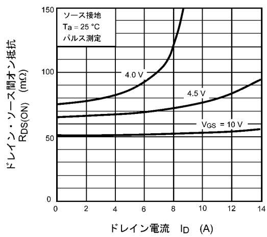
図 7.4 R_{DS(ON)} - I_D
