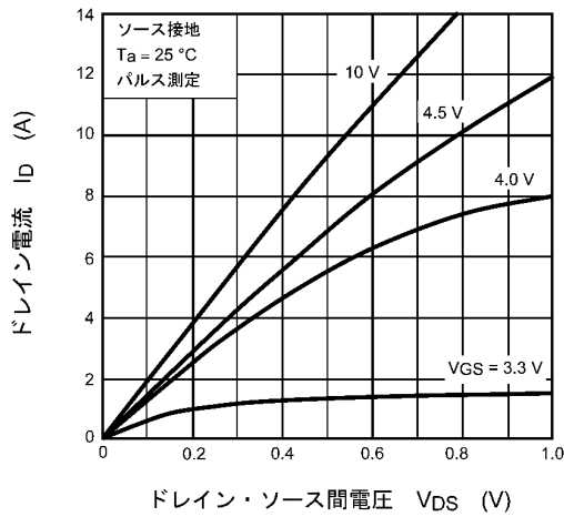
図 7.1 I_D - V_{DS}
