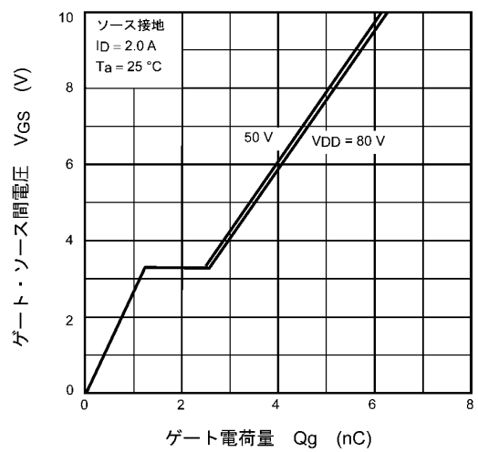
図 7.10 ダイナミック入力特性
