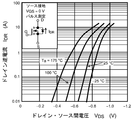
図 7.7 IdR - Vds
