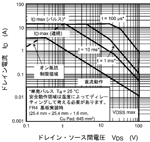
図 7.11 安全動作領域
