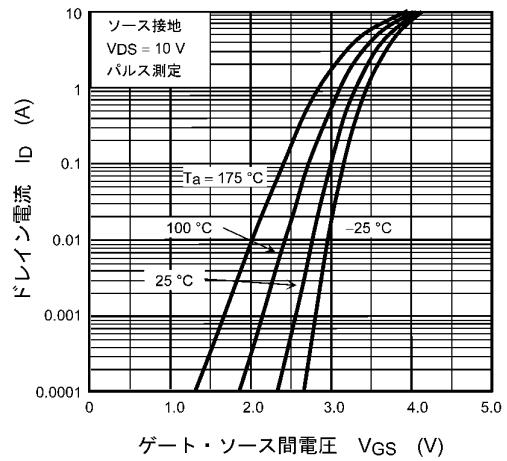
図 7.2 I_D - V_{GS}
