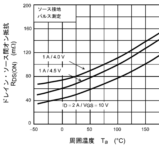
図 7.5 R_{DS(ON)} - T_a
