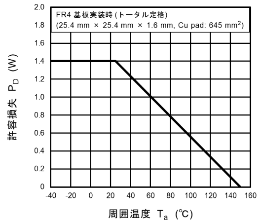
図 7.3.2 P_D - T_a
