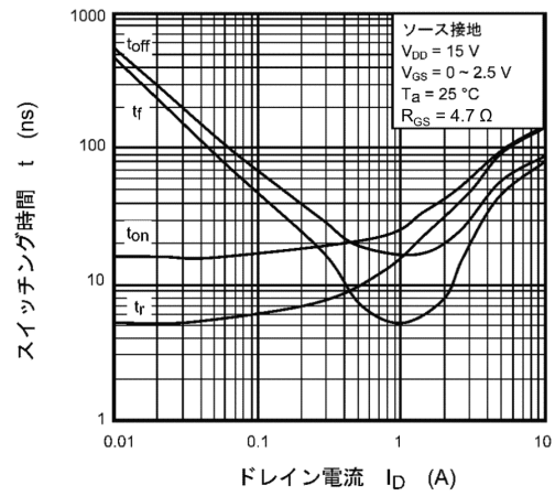
図 7.1.10 t - I_D
