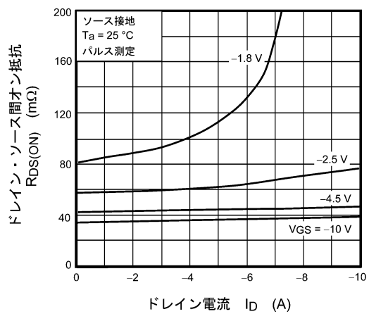
図 7.2.4 R_{DS(ON)} - I_D
