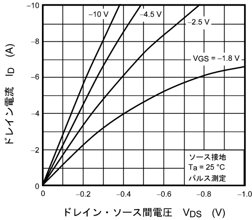
図 7.2.1 I_D - V_{DS}
