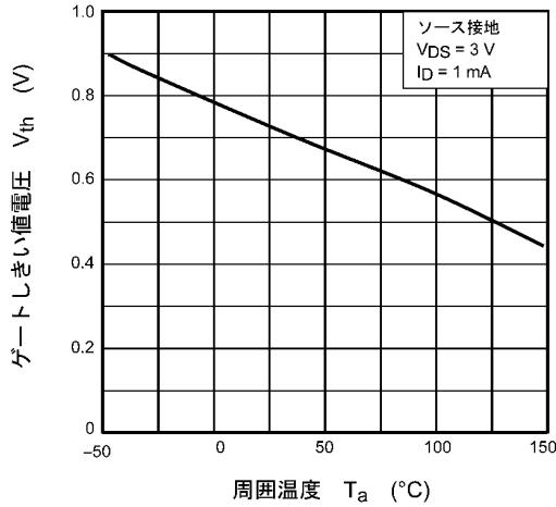
図 7.1.7 V_{th} - T_a
