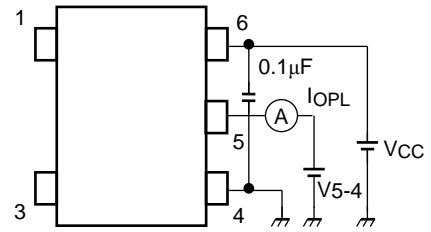
图 2. I OPL 测定回路
