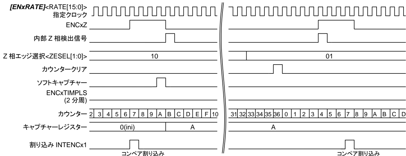
図 3.12 ENCxZ入力無効( [ENxTNCR]\langle ZEN \rangle = 0 )
