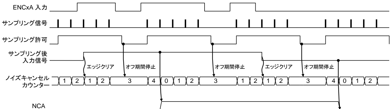
図 3.17 ノイズキャンセル(PWMオン期間サンプリング、PWMオフ期間停止、 \langle NCT[6:0] \rangle = 0x04 )
