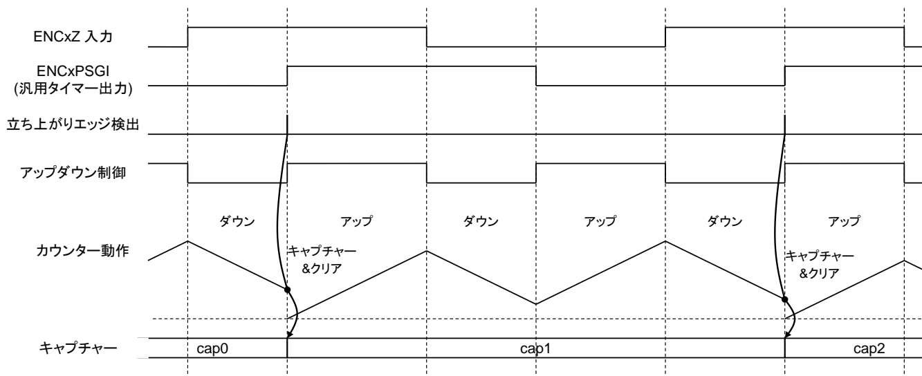
図 3.13 位相カウンターモード(位相差)の動作
