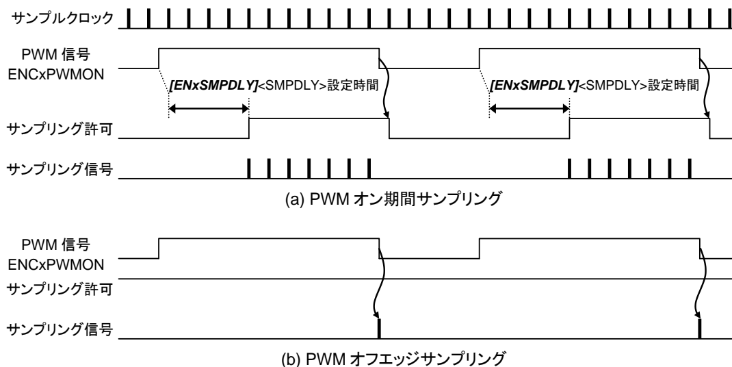
図 3.15 PWM同期サンプリング
