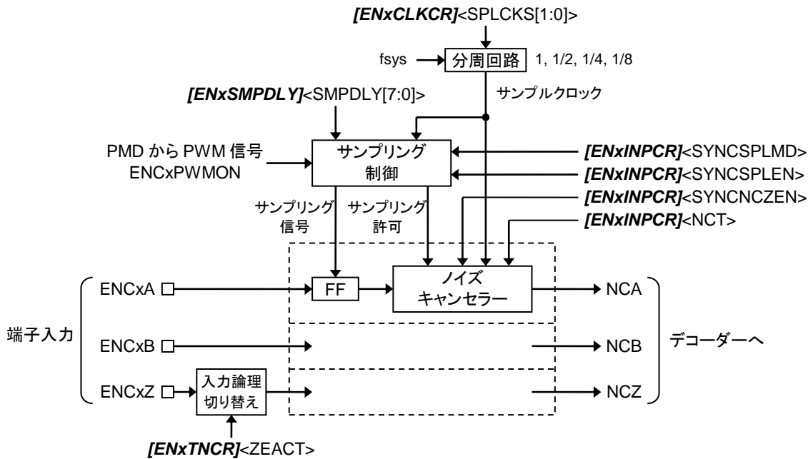
図 3.14 入力回路構成
