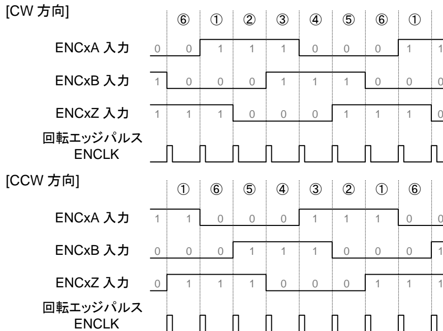
図 3.21 3相デコーダー波形
