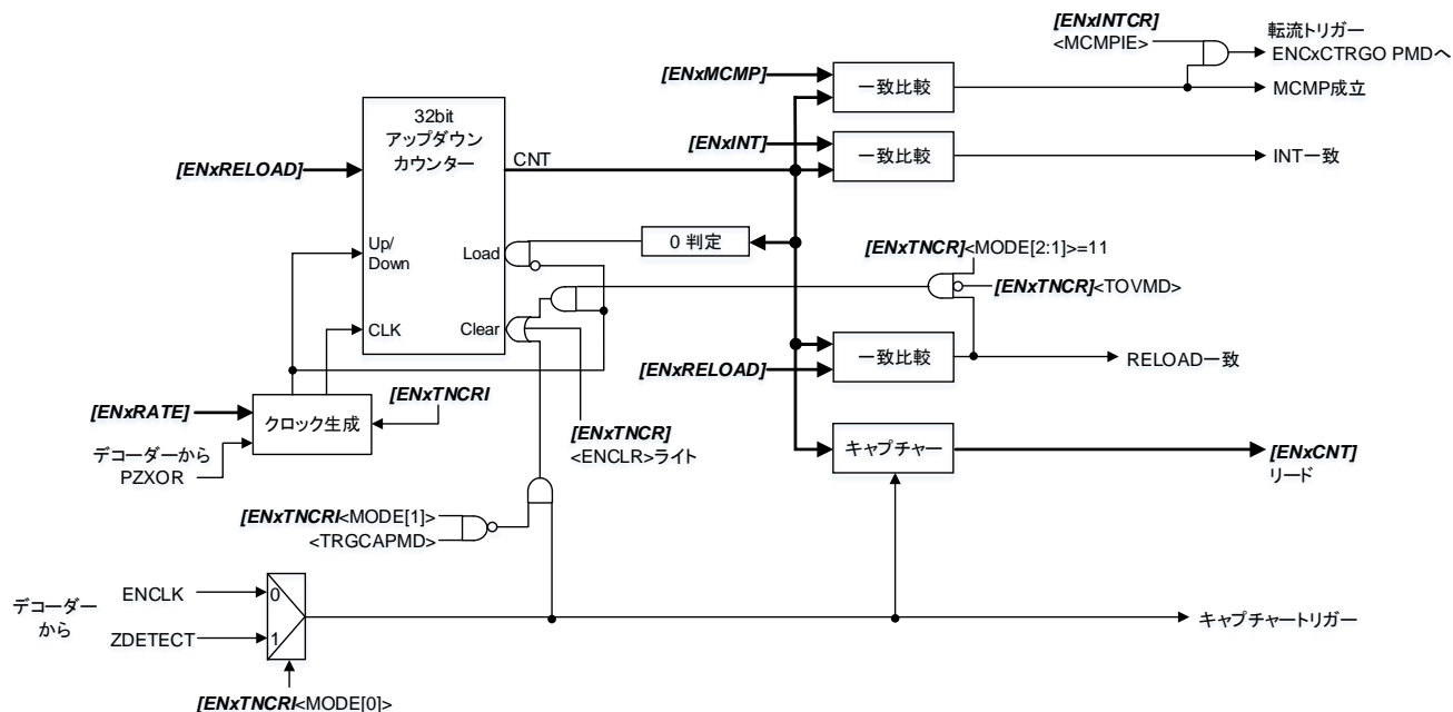
図 3.24 カウンター構成(センサーモード(位相カウント)、位相カウンターモード)
