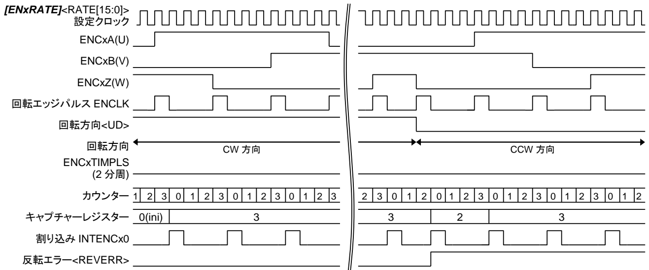
図 3.7 3相デコード( [ENxTNCR] \langle P3EN \rangle = 1 )
