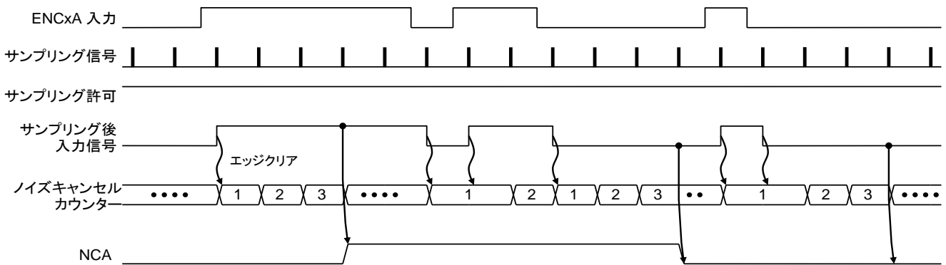
図 3.16 ノイズキャンセル(連続、 \langle NCT[6:0] \rangle = 0x03 )
