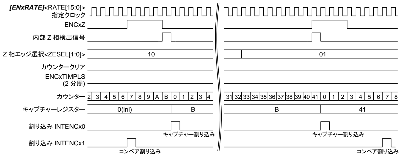
図 3.11 ENCxZ入力有効( [ENxTNCR]\langle ZEN \rangle = 1 )
