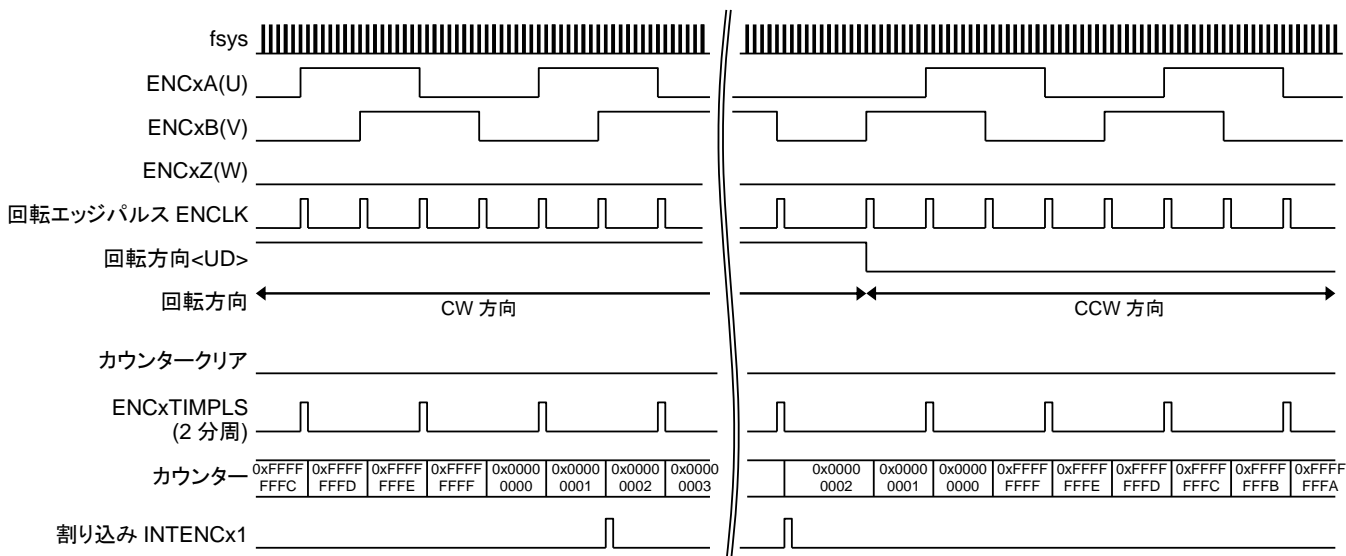
図 3.4 2相デコード( [ENxTNCR]\langle P3EN \rangle = 0 )
