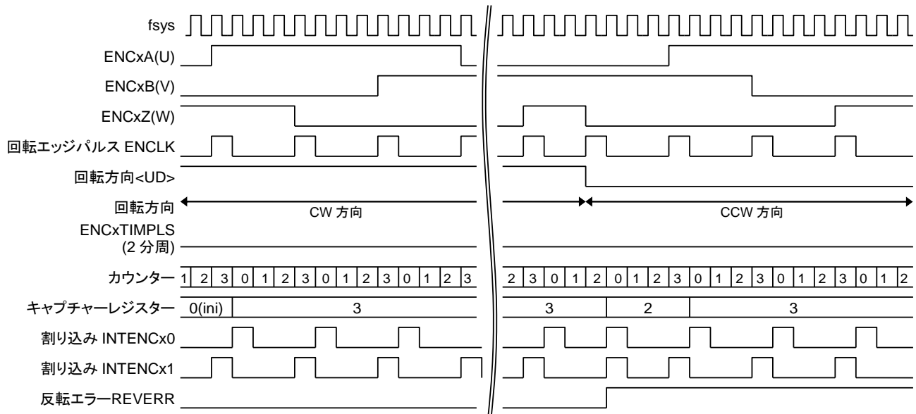
図 3.5 3相デコード( [ENxTNCR] \langle P3EN \rangle = 1 )
