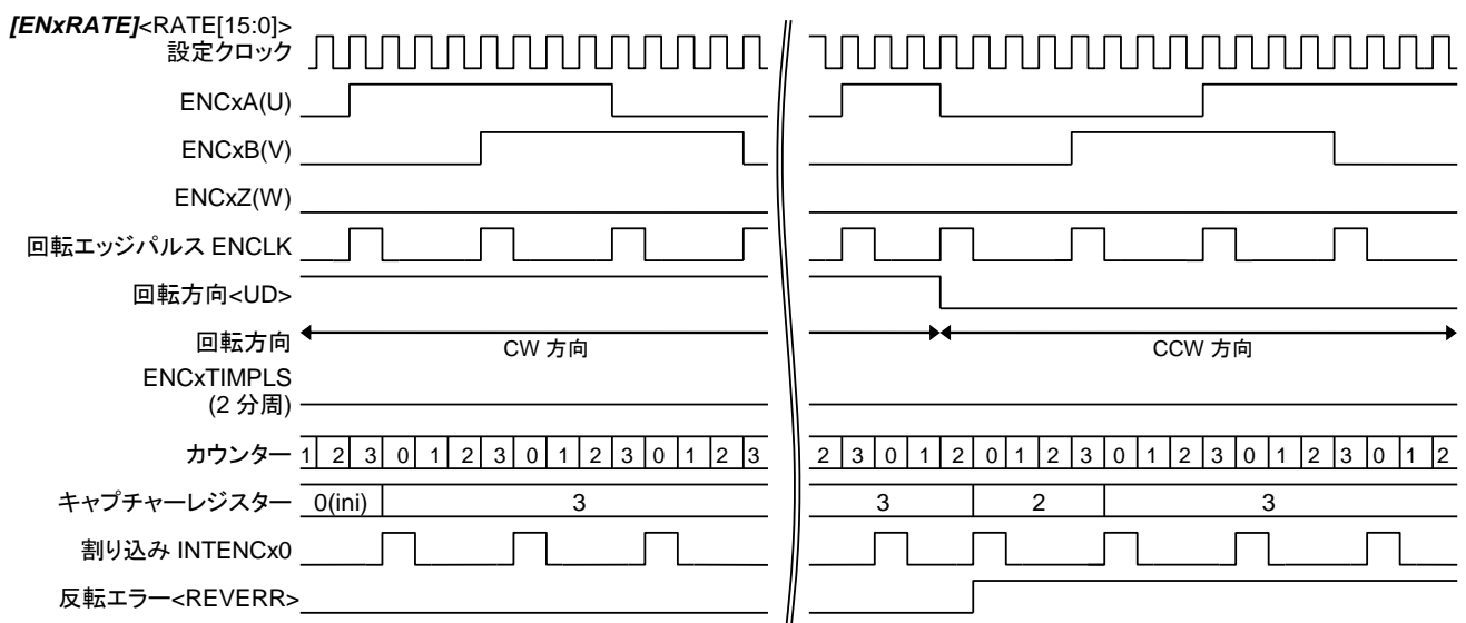
図 3.8 2相デコード( [ENxTNCR] \langle P3EN \rangle = 0 )
