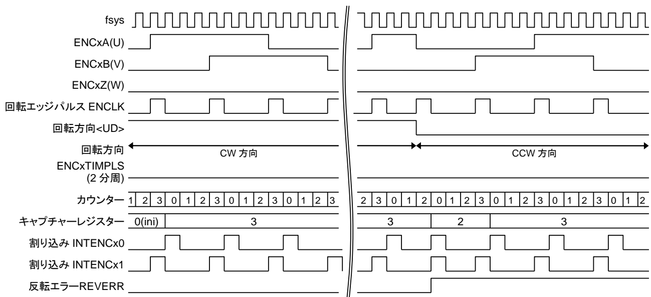
図 3.6 2相デコード( [ENxTNCR] \langle P3EN \rangle = 0 )
