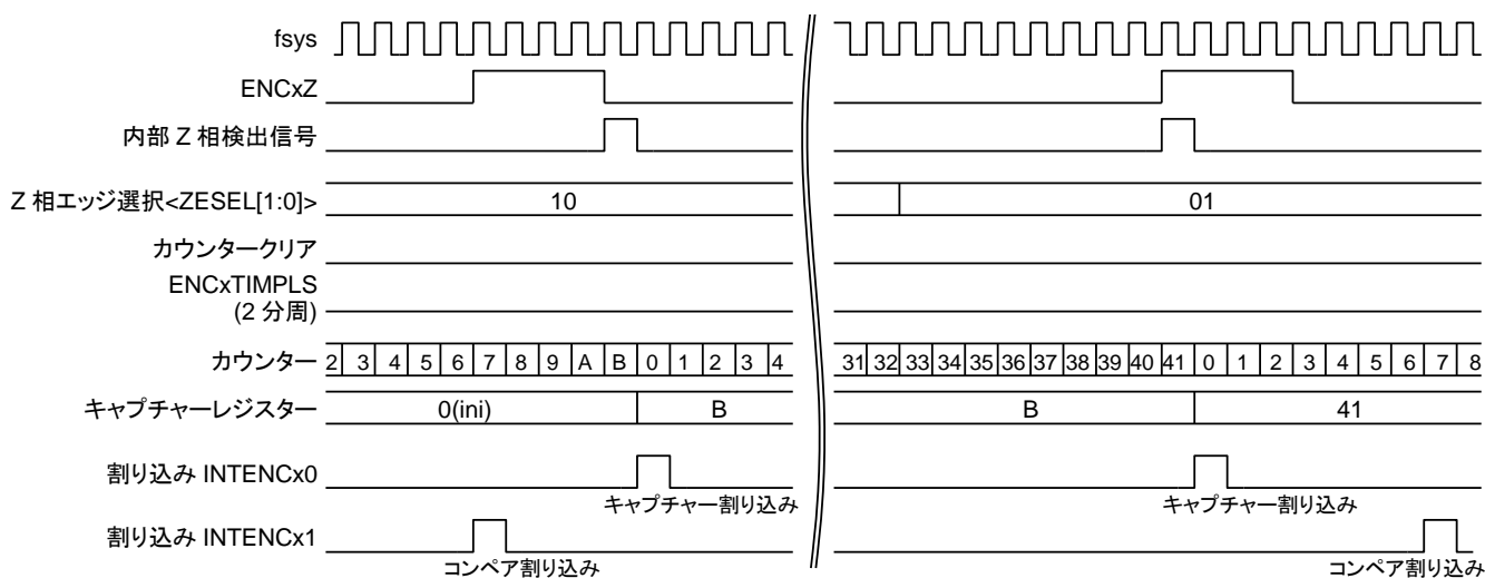
図 3.9 ENCxZ入力有効( [ENxTNCR]<ZEN> = 1 )
