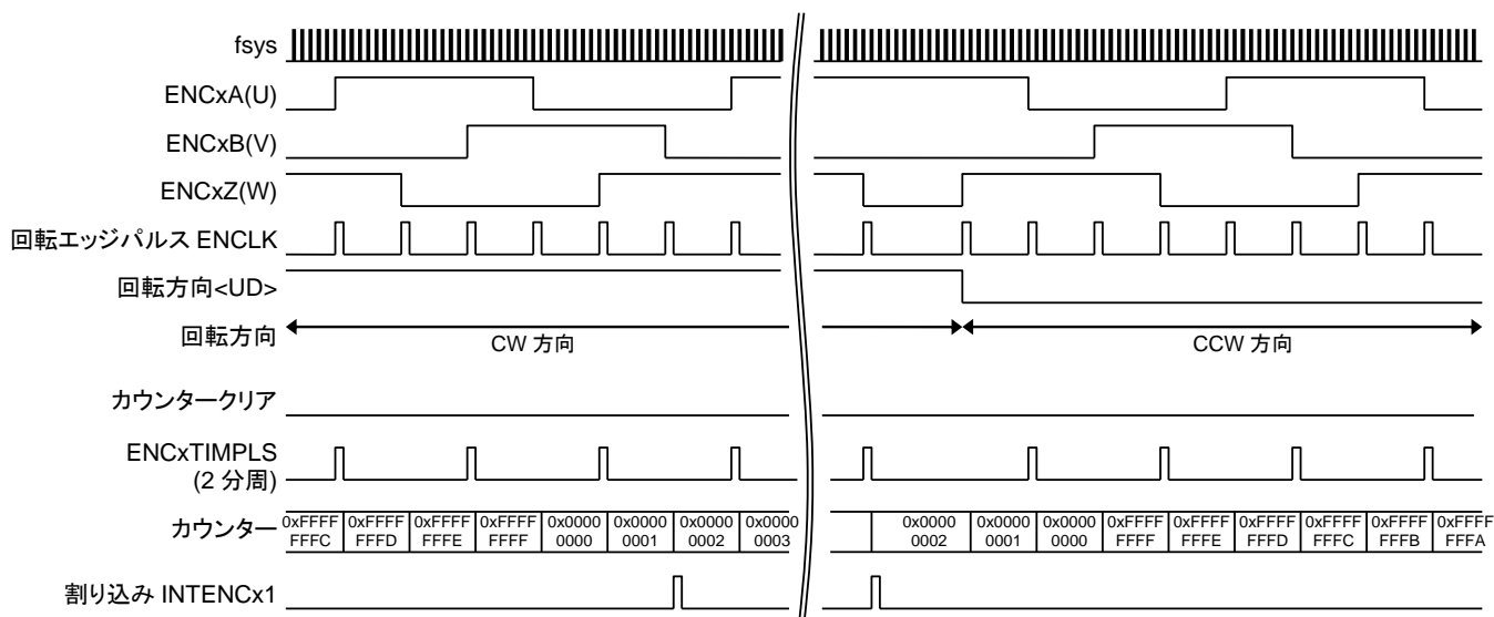
図 3.3 3相デコード( [ENxTNCR] \langle P3EN \rangle = 1 )
