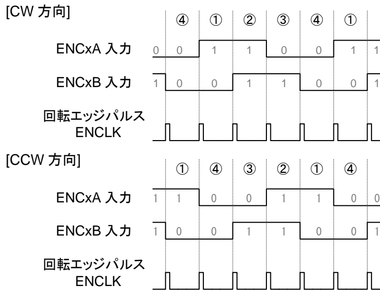
図 3.20 2相デコーダー波形
