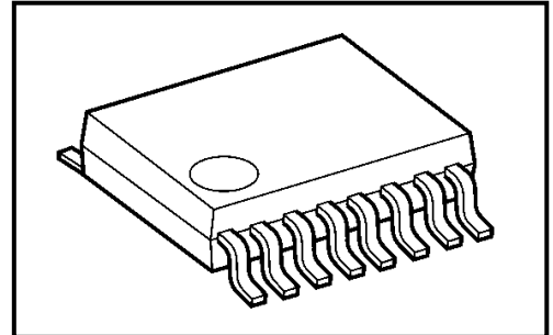
P-TSSOP16-0505-0.65-001 質量 : 0.06 g (typ.)
