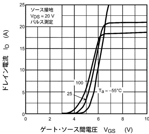
図 8.3 I_D - V_{GS}
