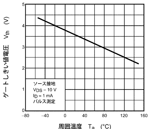
図 8.10 V_{th} - T_a
