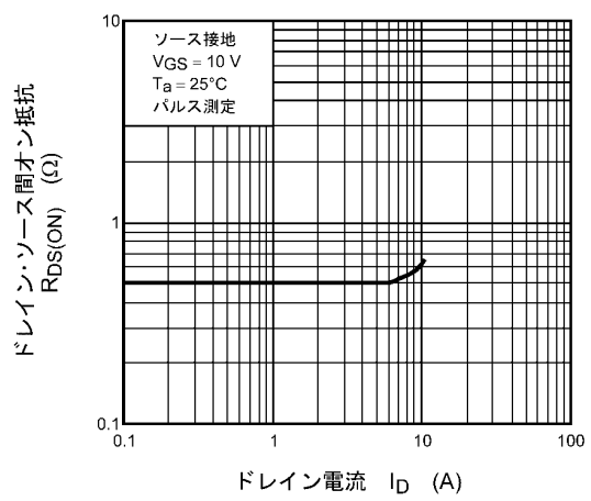
図 8.6 R_{DS(ON)} - I_D
