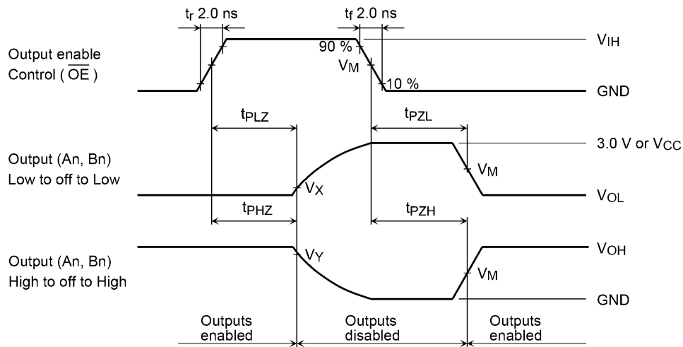
図 14.2 t PLZ , t PHZ , t PZL , t PZH
