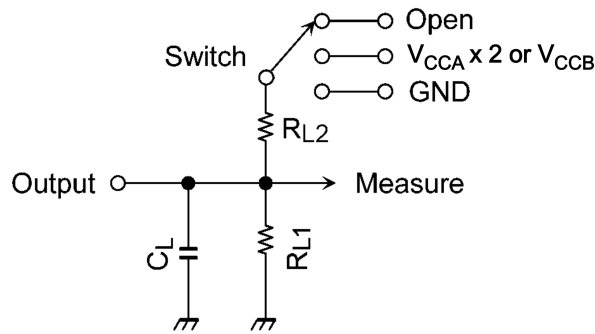
図 13.1 AC電気的特性測定回路
