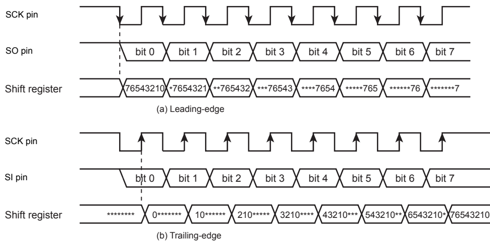
Figure 12-17 Shift Edge
